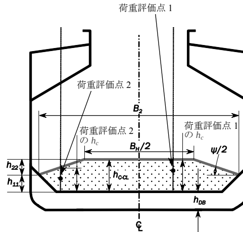
図 4 部分積付の貨物倉における貨物の有効上面の定義 ( h_1 < 0 の場合)
