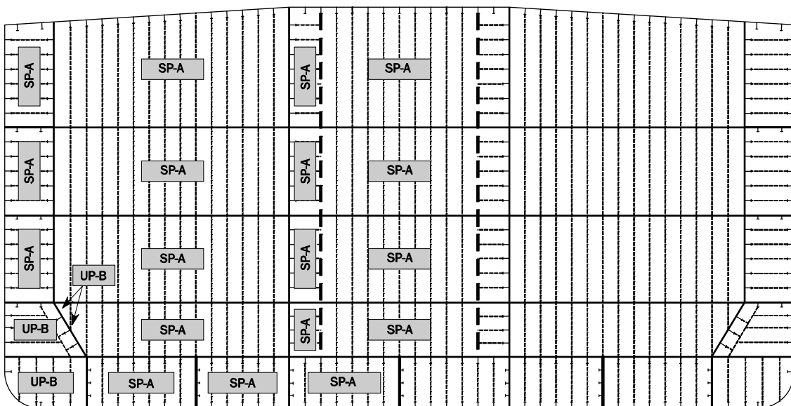
図3 油タンカーの横隔壁
