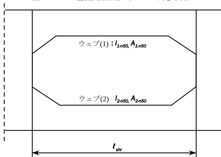
図 14 主要支持部材のウェブの大きな開口
