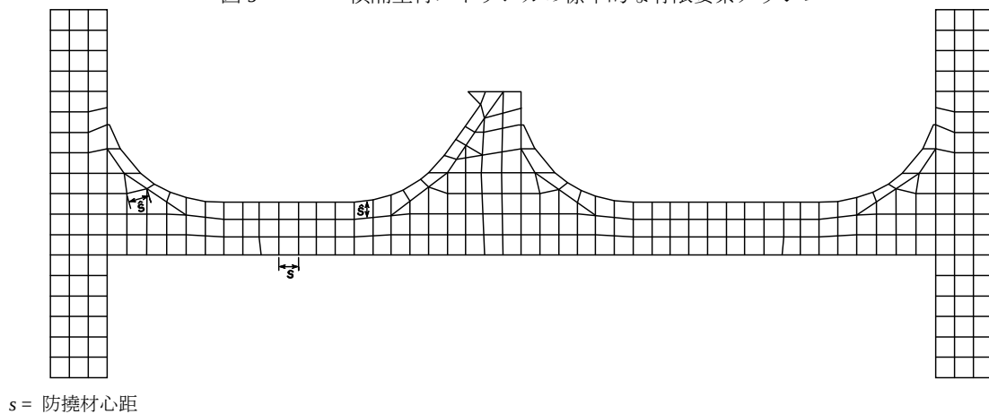
図9 横隔壁付ストリングの標準的な有限要素メッシュ
