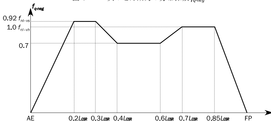
図4 負のせん断力の分布係数 f_{q-neg}
