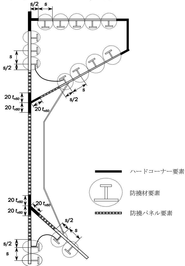
図3 船体横断面の防撓パネル要素、防撓材要素及びハードコーナー要素の配置例
