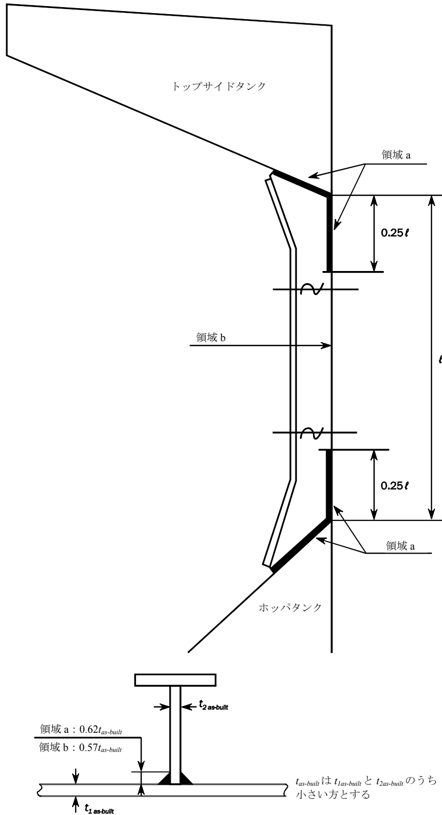
図 11 ばら積運搬船の倉内肋骨
