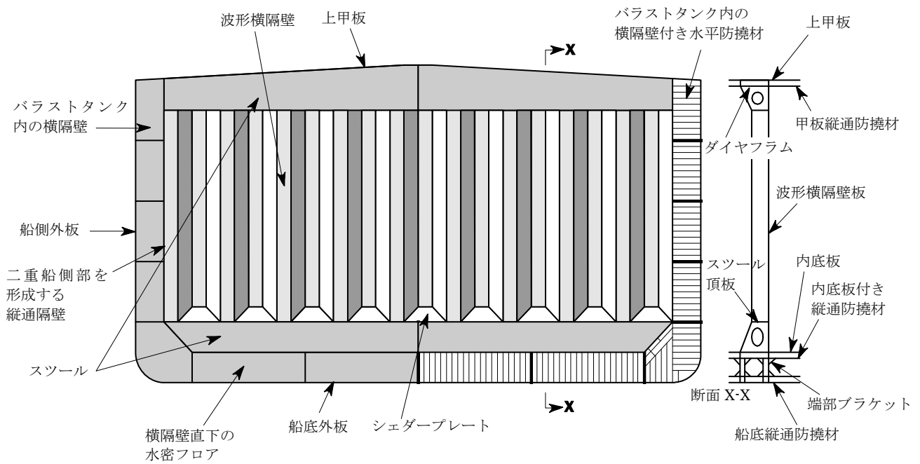
図 4 二重船殻タンカーの波形隔壁
