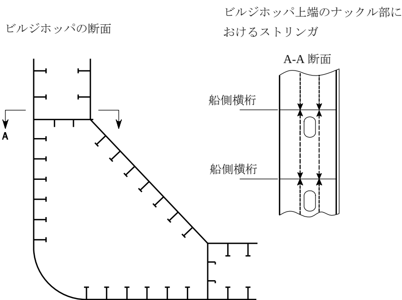
図1 ナックル部の補強例
