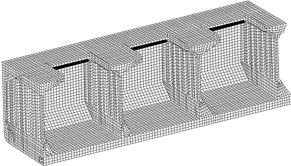
図 4 ばら積貨物船の中央部区域内における 3 ホールドモデルの例
