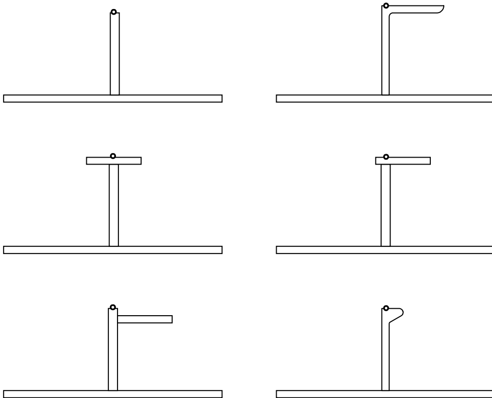
図 24 局局部材寸法評価のための断面係数及びハルガード応力の計算における基準点
