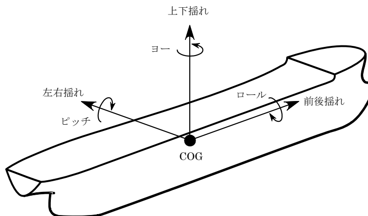
図1 船体運動の正方向の定義
