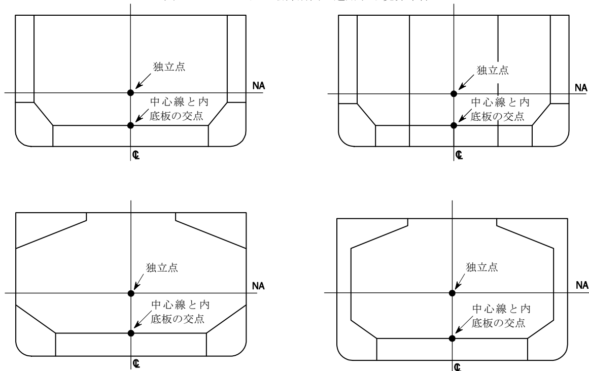
図 17 モデル端部断面に適用する境界条件
