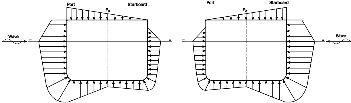
図6 荷重ケース BSP-1P (左) 及び BSP-1S (右) における船体中央での動圧の横方向分布
