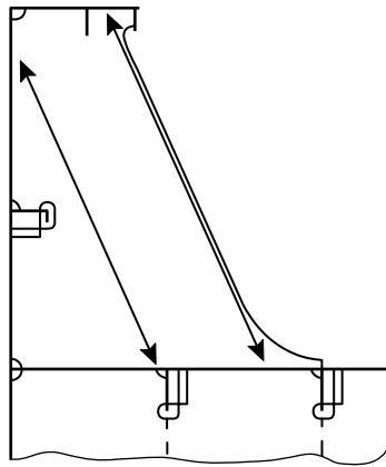
図 2 ハッチコーミングステイ (例 1)
