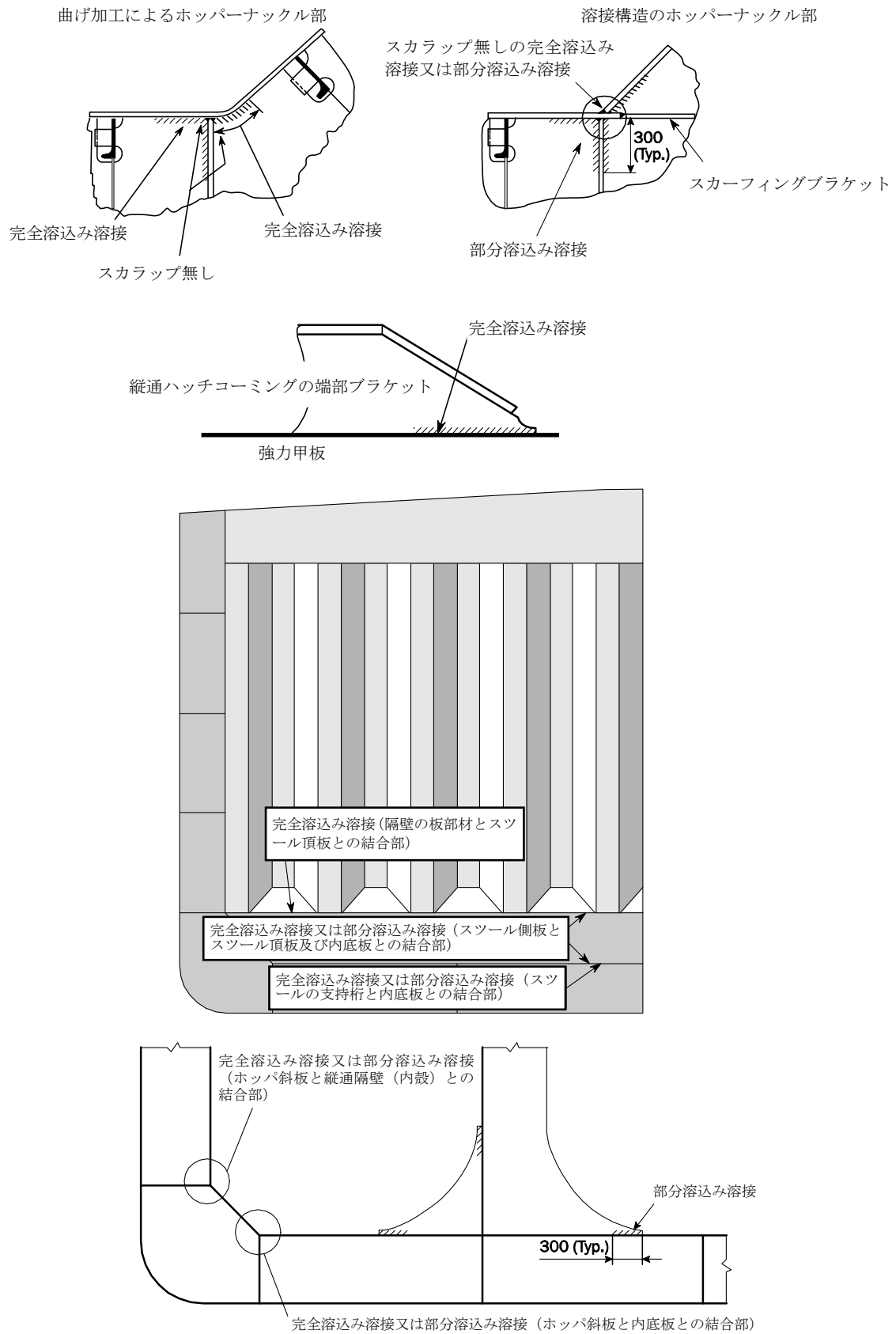
図3 溶接部の高応力域 (例)
