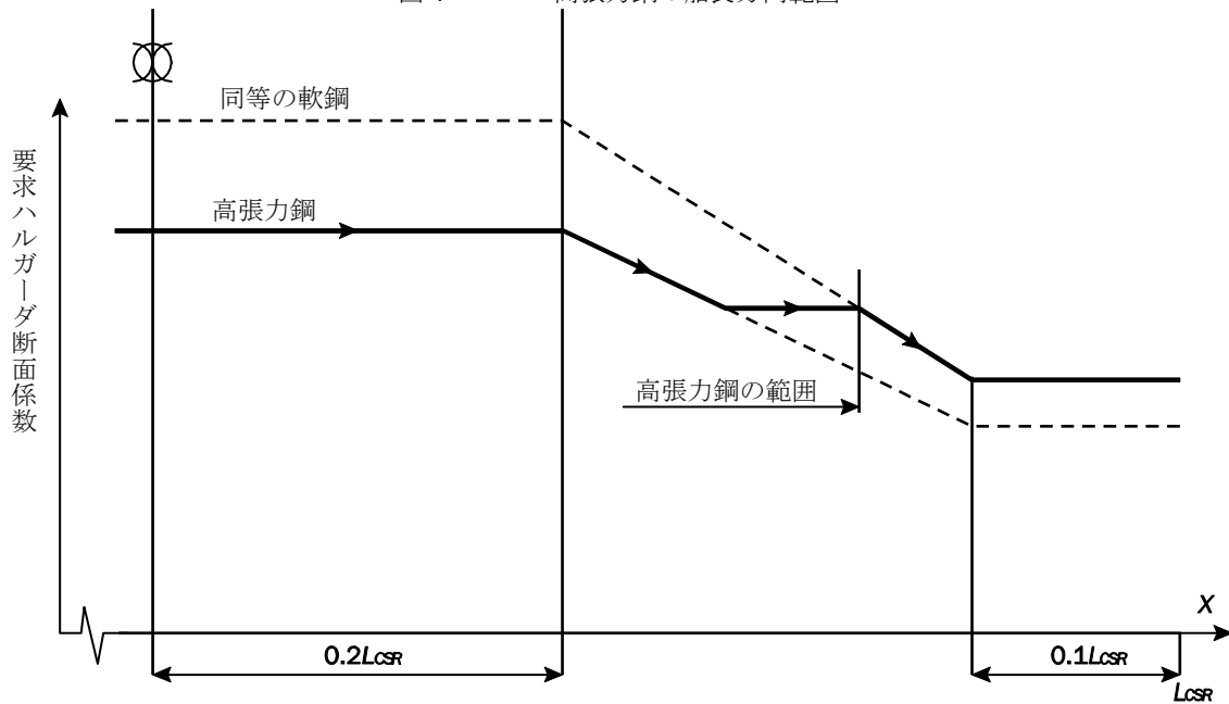
図4 高張力鋼の船長方向範囲
