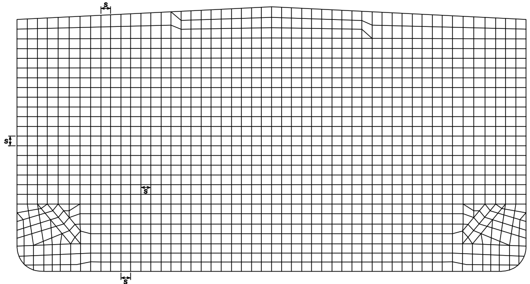
図 8 横隔壁の標準的な有限要素メッシュ
