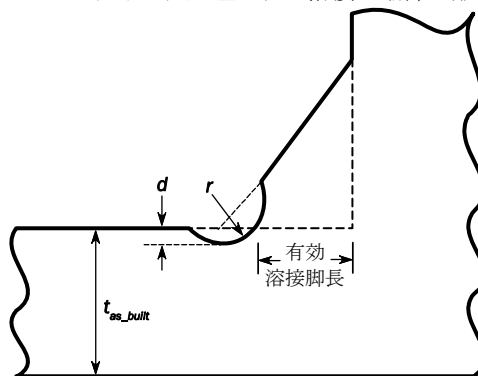
図 5 グラインダ処理された溶接止端部の形状の詳細
