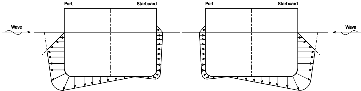
図8 荷重ケース OST-1P (左) 及び OST-1S (右) における船体中央での動圧の横方向分布
