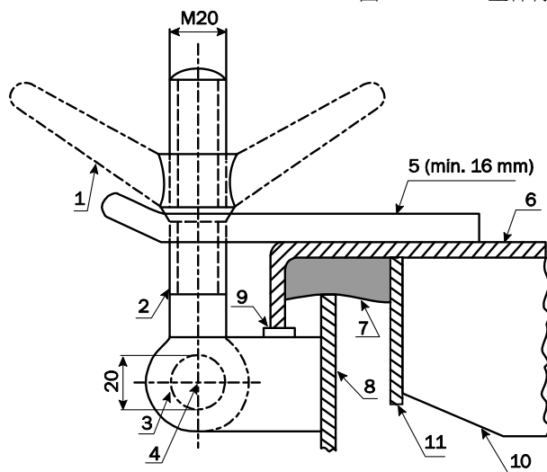
図 1 主締付装置の例
