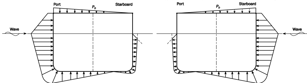
図9 荷重ケース OST-2P (左) 及び OST-2S (右) における船体中央での動圧の横方向分布
