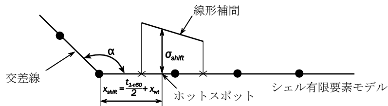
図 19 桁等で支持された十字継手のホットスポット応力の算出手順
