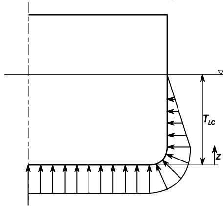
図 1 静水圧 P_S
