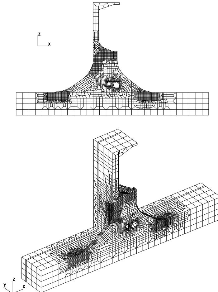
図 16 隔壁と二重底構造間のバットレス結合部の解析に用いる局部モデルの例 (左舷側半分を図示する)
