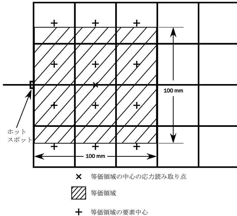
図 25 50 \times 50 \text{ mm} 未満の要素サイズに対する等価領域
