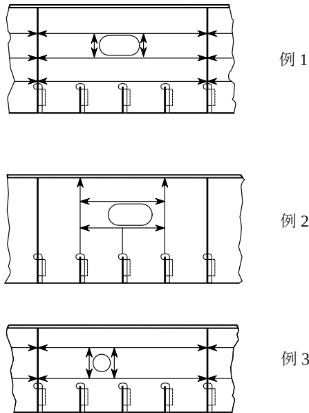
図 13 開口を有するウェブ
