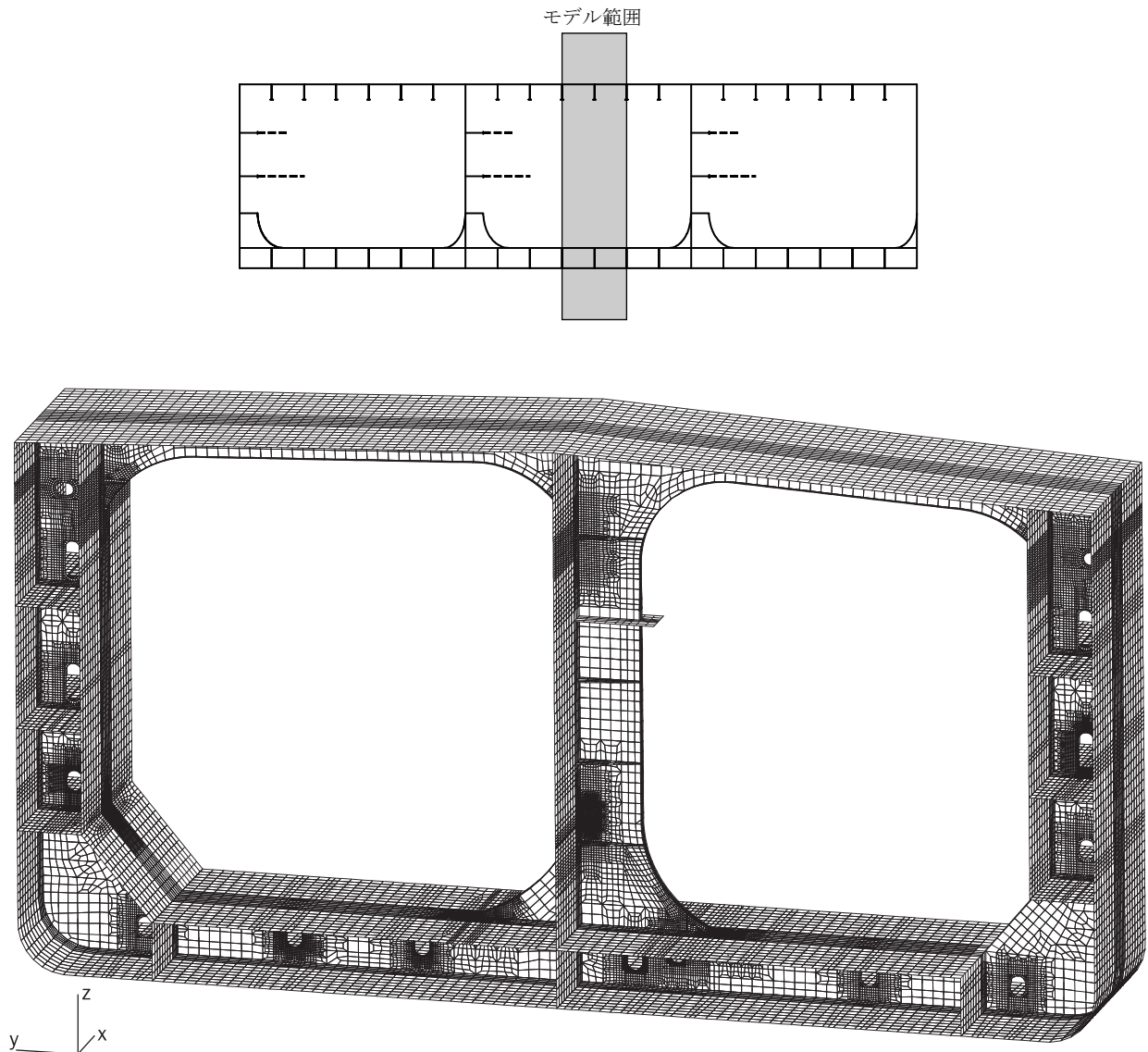
図 11 横桁結合部及び開口部の詳細メッシュ解析に用いる局部モデルの範囲の例
