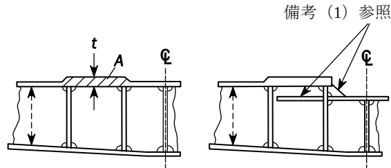
図1 機器の台座 タイプ1
