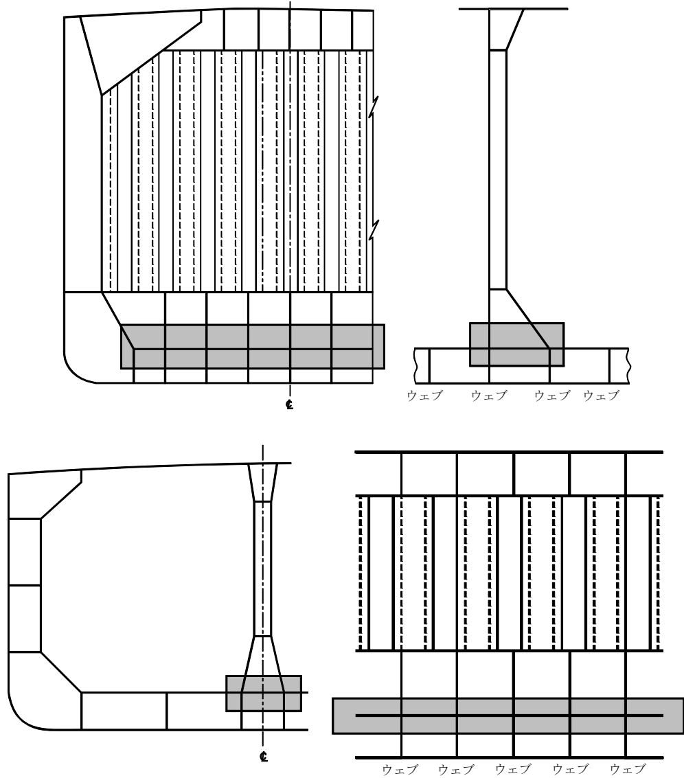
図 5 下部スツールと内底板及びホップタンク斜板との結合部におけるスクリーニング箇所
