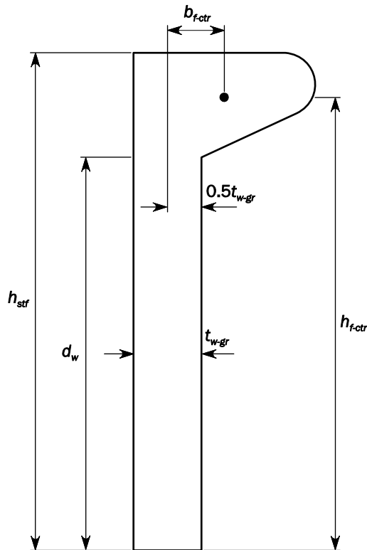
図 15 バルブプレートの特性
