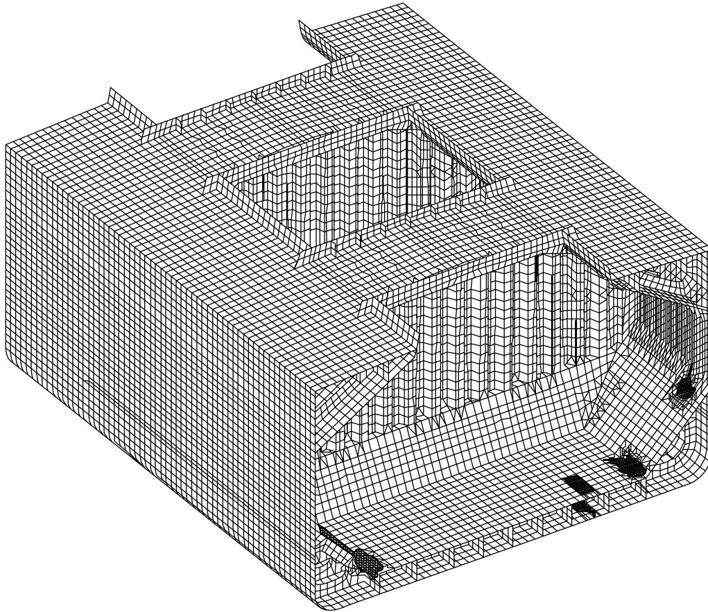
図2 貨物倉モデルに直接組み込まれた極詳細メッシュ領域
