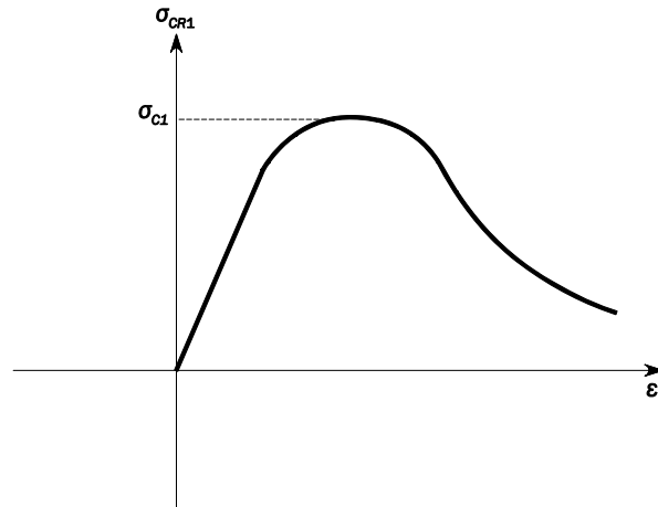
図 8 梁柱座屈に対する応力-ひずみ曲線 \sigma_{CR1} - \varepsilon
