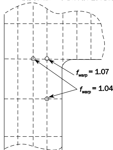
図 1 ばら積貨物船の甲板付縦通防撓材のそり影響
