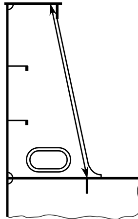
図 5 ハッチコーミングステイ (例 4)
