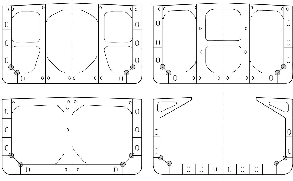
図1 二重船側を有する船のホッパナックル部における必須評価箇所
