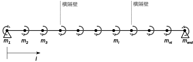
図 19 中央部貨物倉区域以外における曲げモーメントの調整
