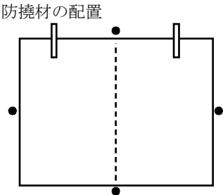
呼び寸法 630×830
