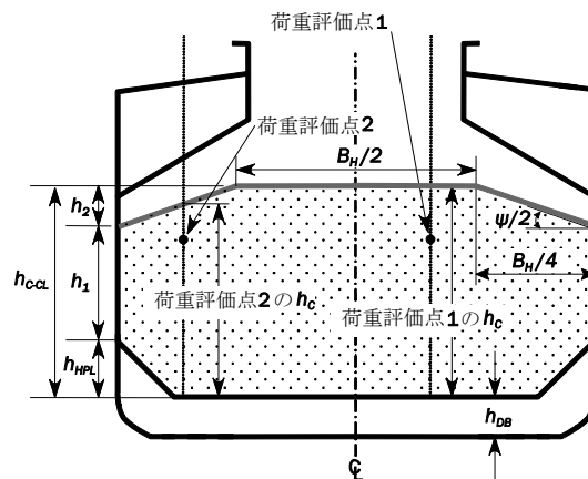
図3 部分積付の貨物倉における貨物の有効上面の定義 ( h_1 \geq 0 の場合)
