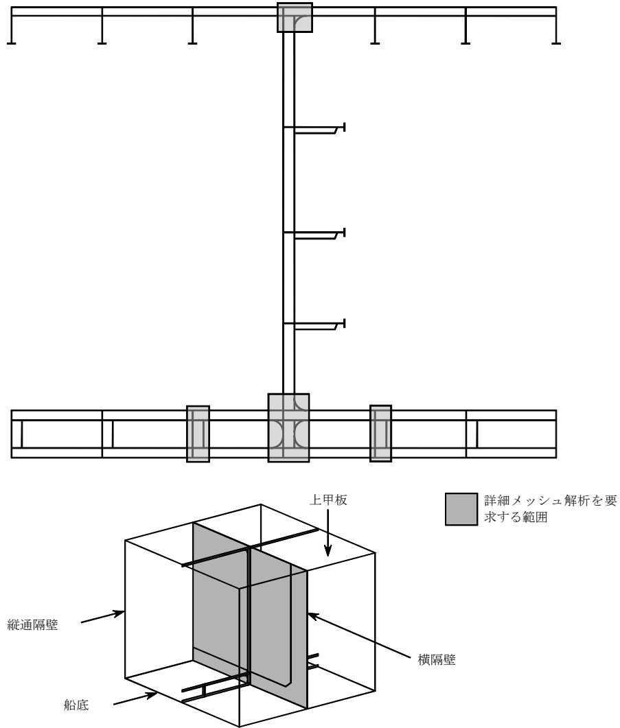
図3 二重底又は上甲板の縦通防撓材と横隔壁周辺構造との結合部における評価必須箇所例
