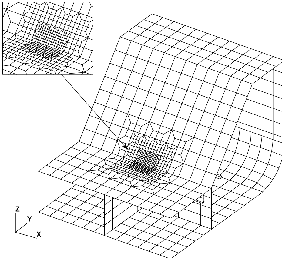
図3 内底板とビルジホッパ斜板とのナックル結合部の局部極詳細メッシュモデル( t_{n50} \times t_{n50} )
