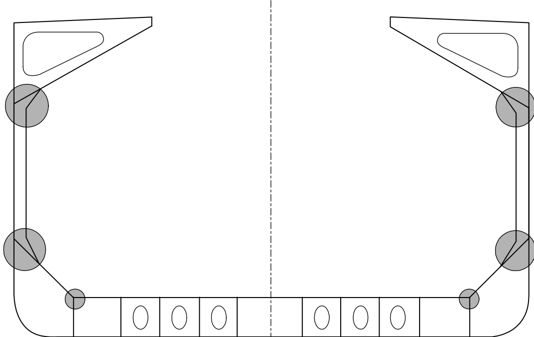
図2 単船側ばら積貨物船の上部ナックル部，倉内肋骨の上部及び下部端部ブラケットにおける必須評価箇所
