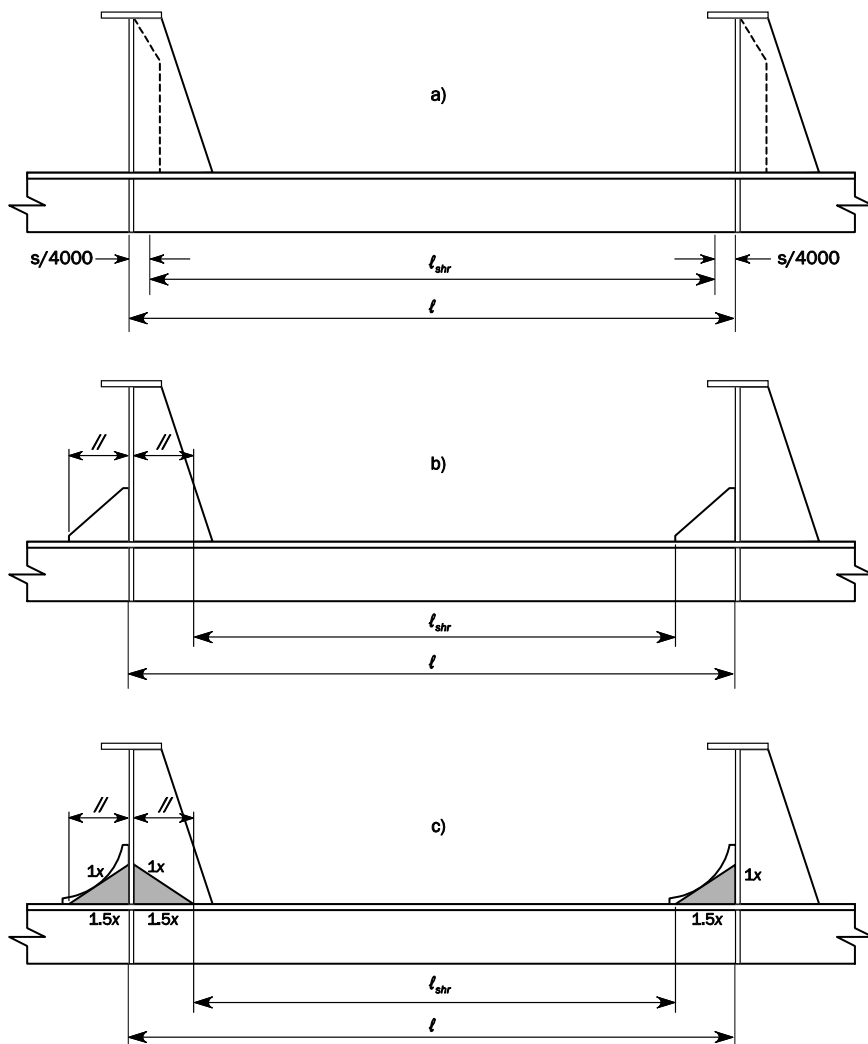
図4 ウェブ防撓材に支持される防撓材有効せん断スパン（単船殻構造）
