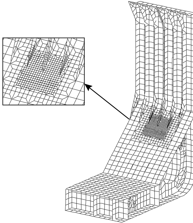
図 10 倉内肋骨のブラケットの局部有限要素モデル, t_{n50} \times t_{n50} メッシュ
