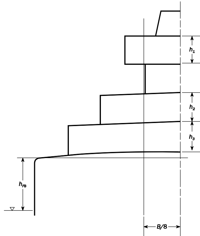
図 1 甲板室の有効高さ
