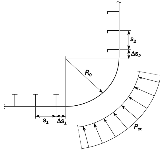
図 1 横式構造のビルジ外板
