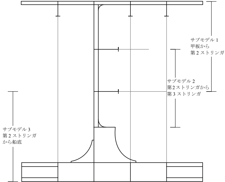
図 14 局部モデルを用いた横隔壁構造の局部解析の例
