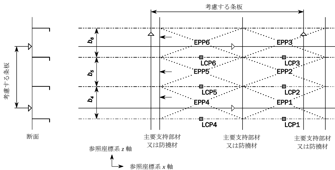
図 19 縦式構造における荷重計算点 (LCP)
