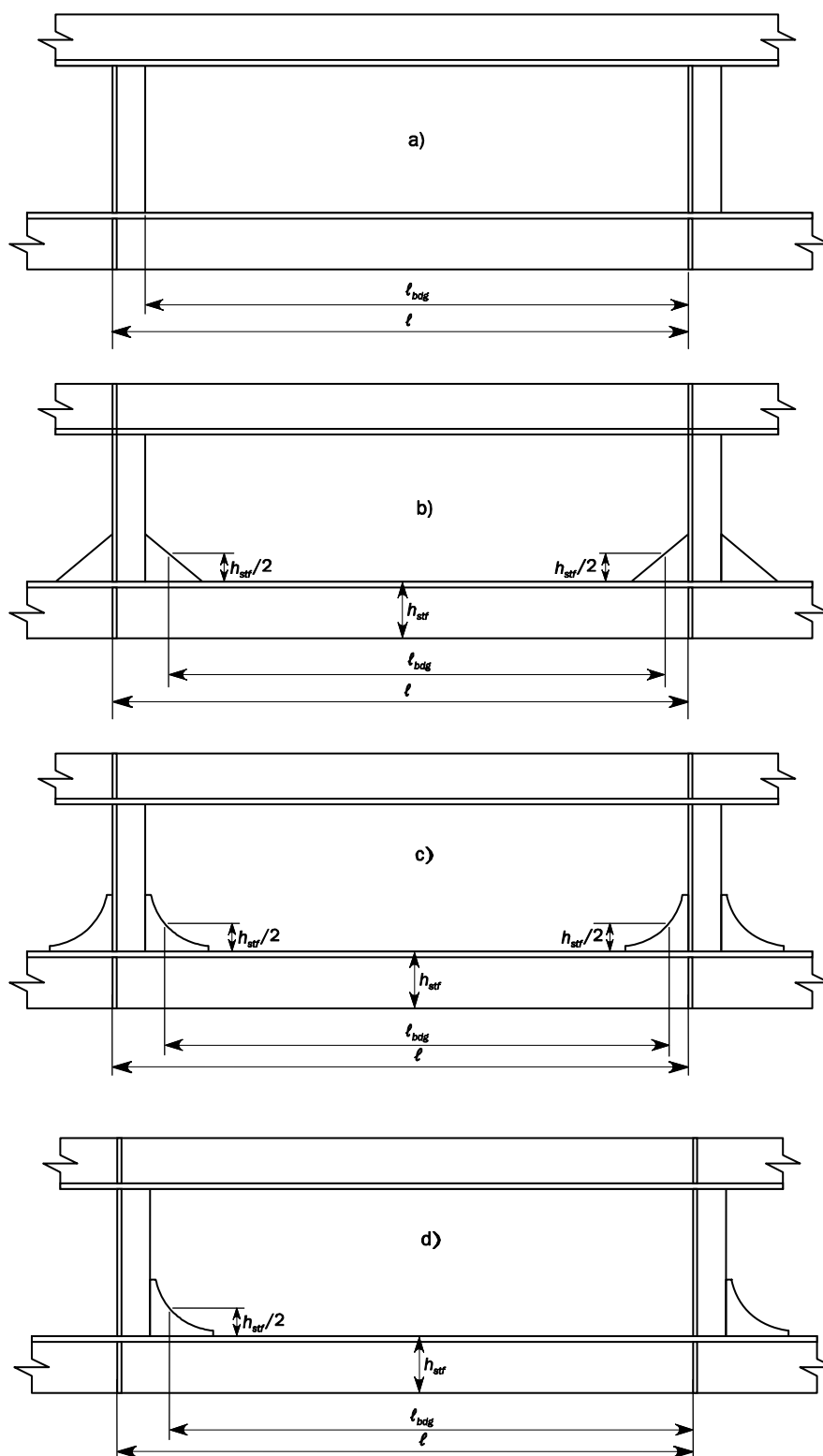
図2 ウェブ防撓材に支持される防撓材の有効曲げスパン（二重殻構造）
