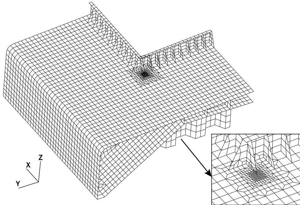
図 12 ハッチサイドコーミング端部ブラケットと甲板との結合部の 極詳細メッシュ局有限要素モデル, t_{n50} \times t_{n50} メッシュ
