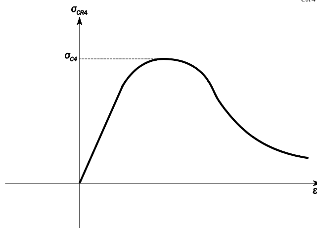
図 10 ウェブの局部座屈に対する応力-ひずみ曲線 \sigma_{CR4} - \varepsilon
