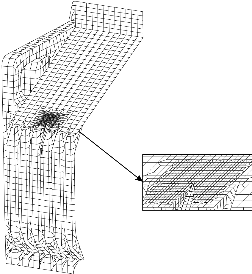
図 11 倉内肋骨の上部ブラケットの局部有限要素モデル, t_{n50} \times t_{n50} メッシュ
