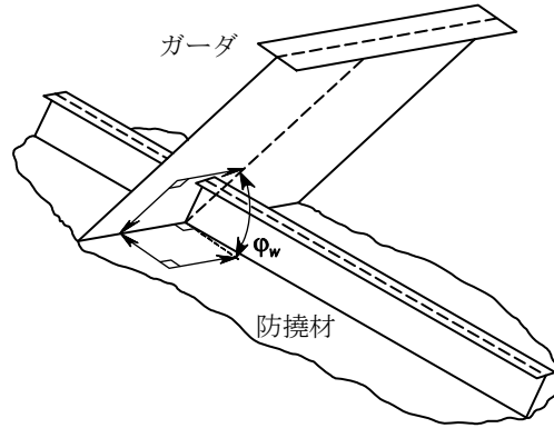
図5 外板付き主要支持部材と外板のなす角度
