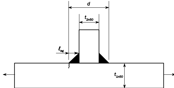
図 2 十字継手、T 字継手及び横方向の付加物継手の溶接止端部の距離
