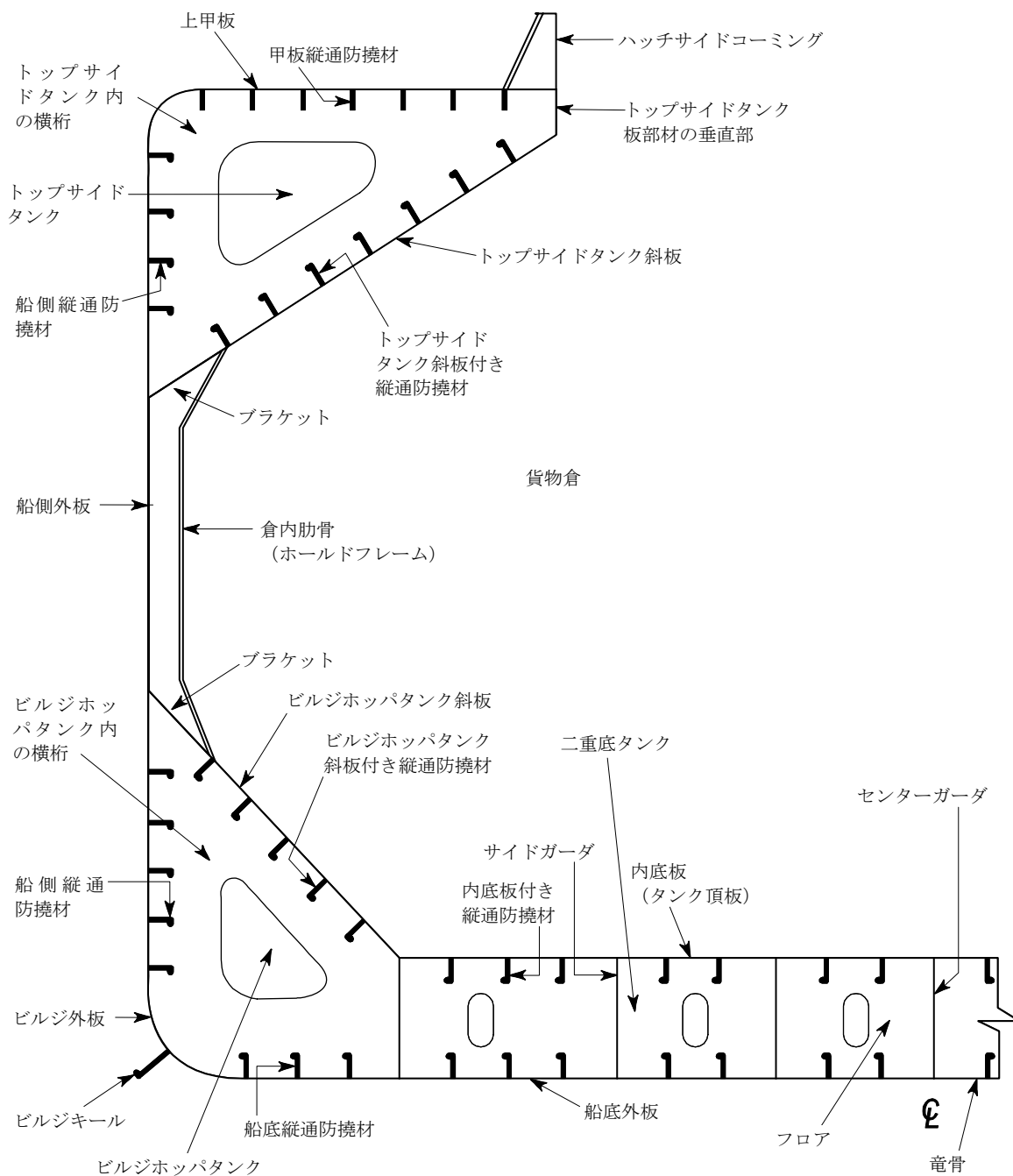
図 7 単船側ばら積貨物船の中央部貨物倉の横断面
