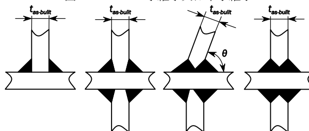
図 1 T 字継手又は十字継手
