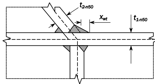
図 18 桁等で支持された十字継手の板厚等の定義
