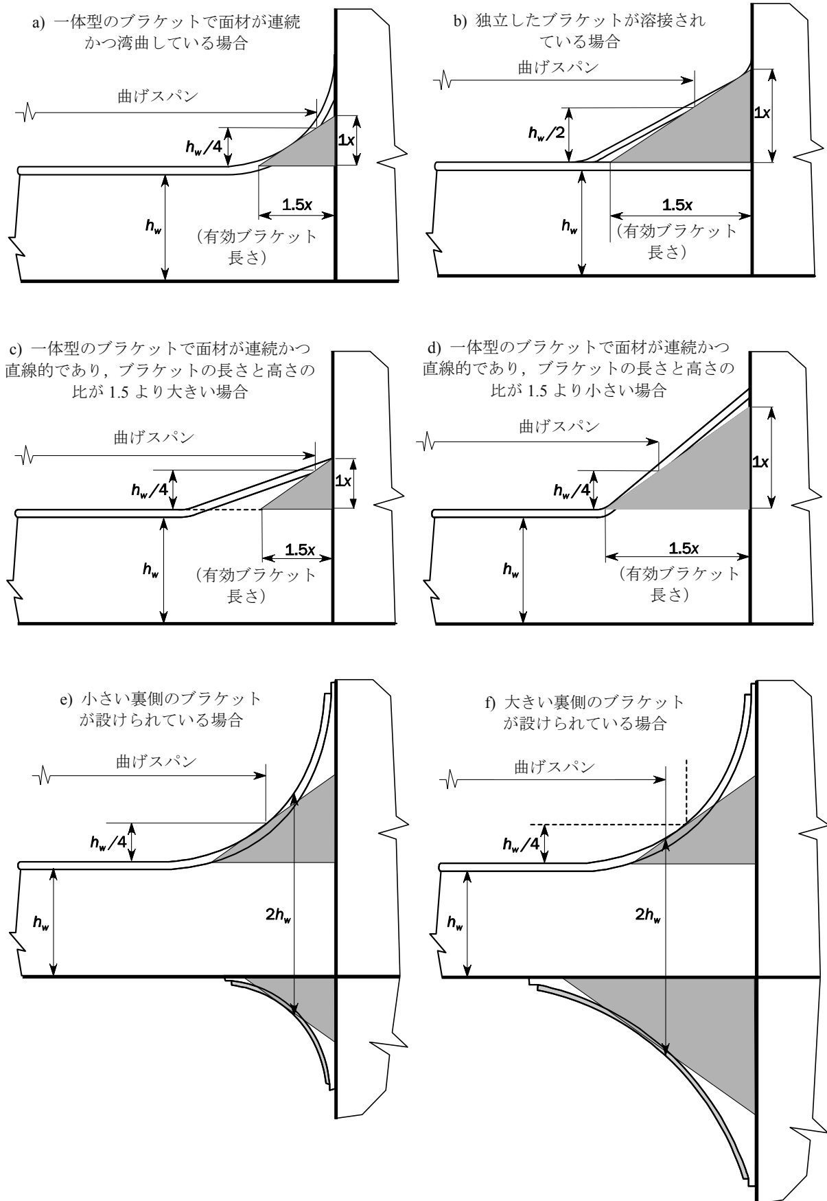
図9 主要支持部材の有効曲げスパン
