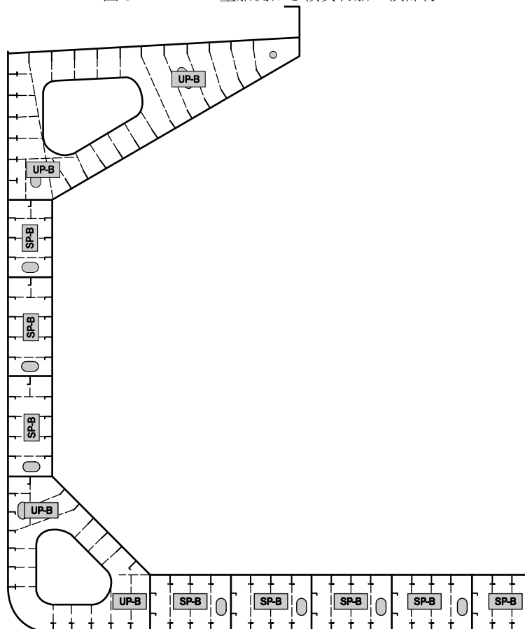
図 8 二重船側ばら積貨物船の横部材
