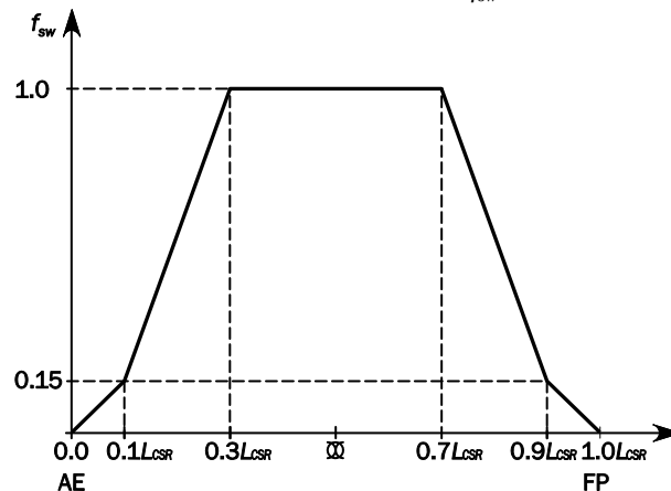
図 1 分布係数 f_{sw}
