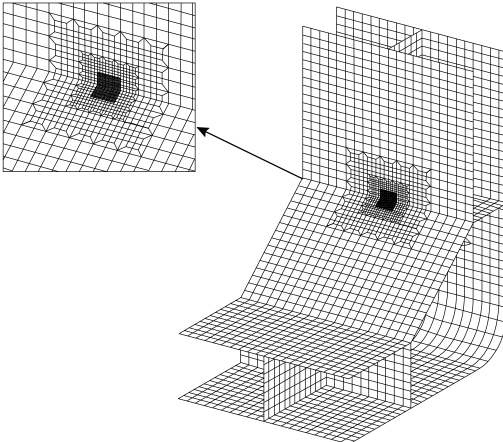
図5 二重船殻縦通隔壁とビルジホップ斜板との上部ナックル結合部の局部極詳細メッシュモデル( t_{n50} \times t_{n50} )
