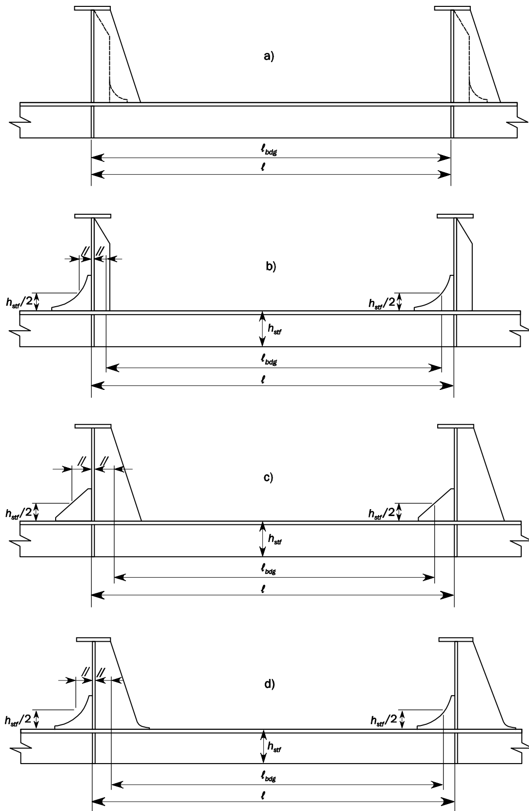
図1 ウェブ防撓材に支持される防撓材の有効曲げスパン（単船殻構造）
