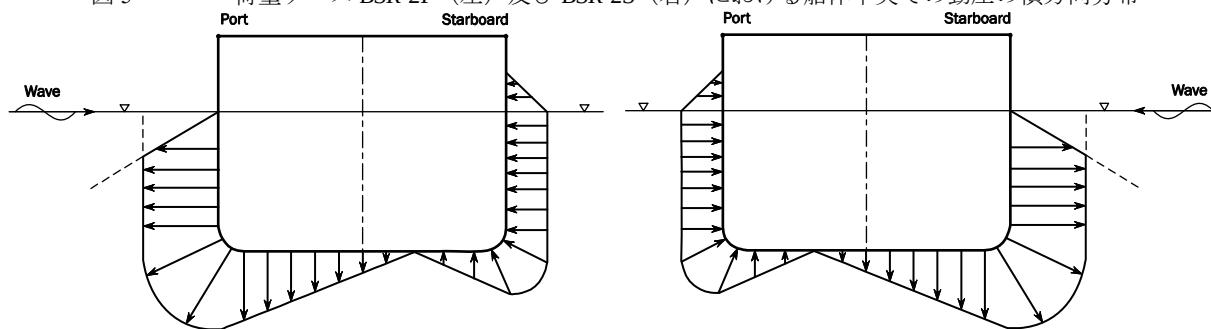
図 5 荷重ケース BSR-2P (左) 及び BSR-2S (右) における船体中央での動圧の横方向分布
