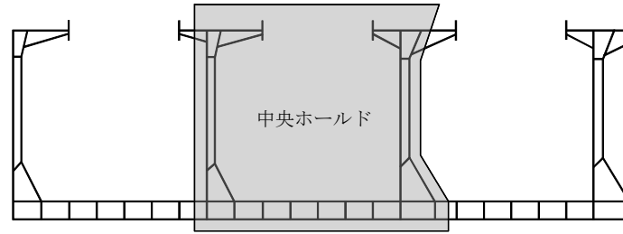
図 22 ばら積貨物船の船長方向の評価範囲
