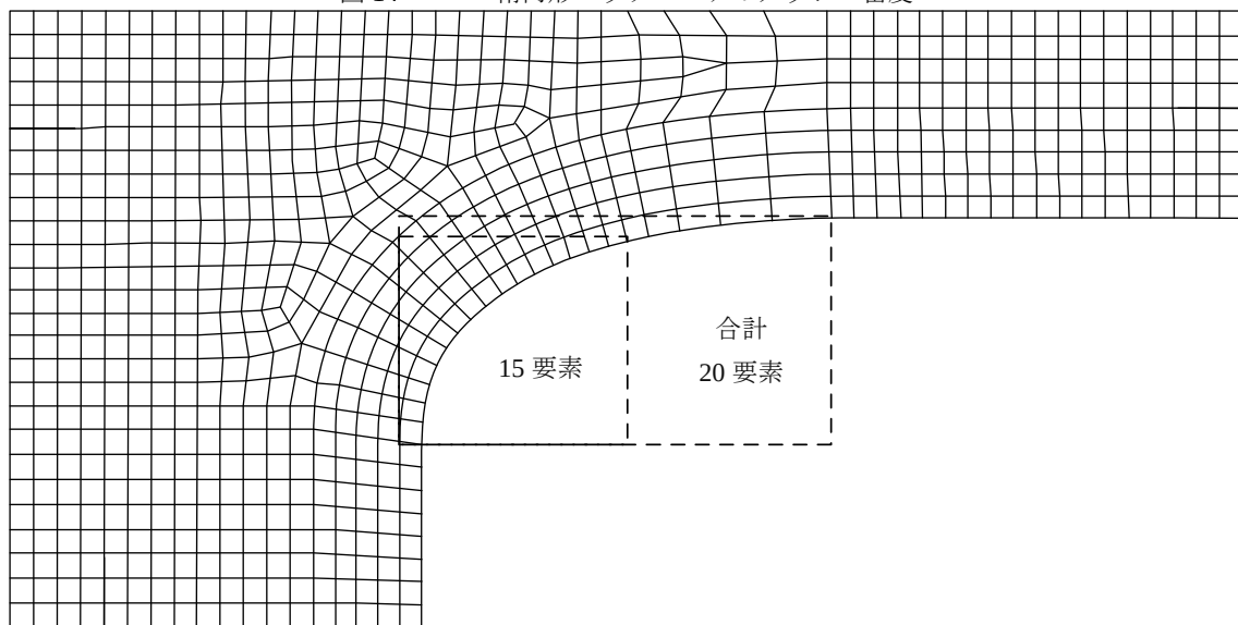
図 14 楕円形ハッチコーナのメッシュ密度
