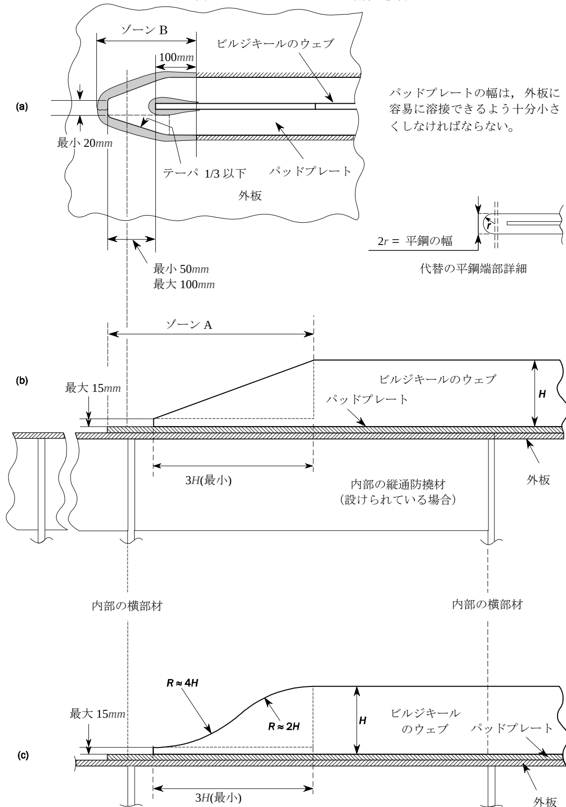
図 19 ビルジキールの端部の設計
