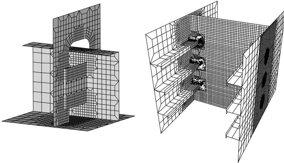
図 1 等価設計の検証に用いる有限要素モデル
