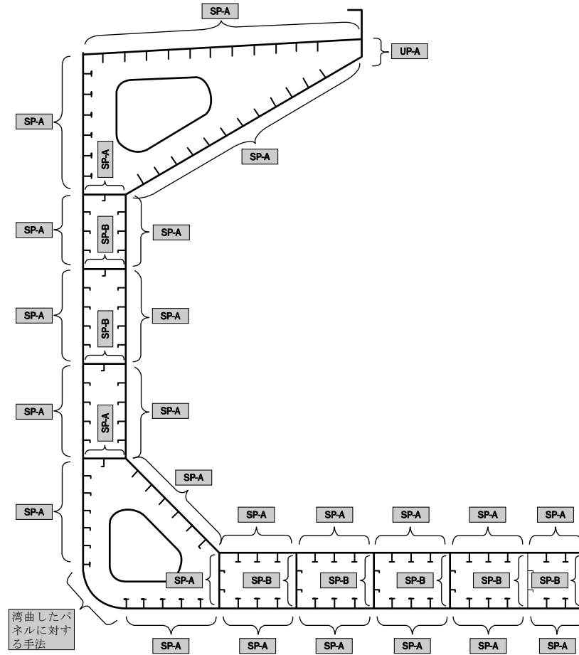
図 7 二重船側ばら積貨物船の縦通板部材
