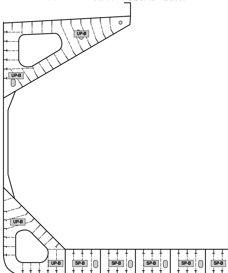
図6 単船側ばら積貨物船の横部材
