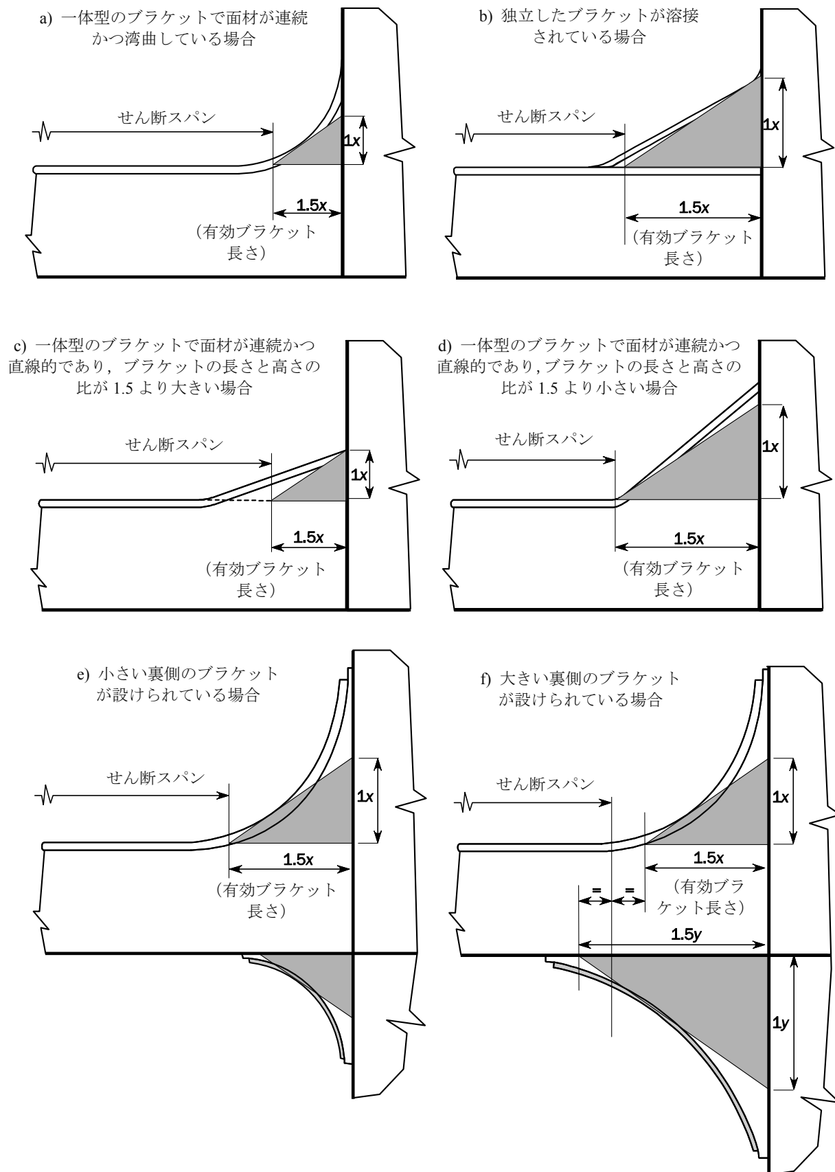
図 10 主要支持部材の有効せん断スパン
