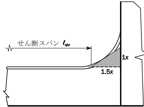
図6 面材がブラケットに沿って連続する局部支持部材の有効せん断スパン
