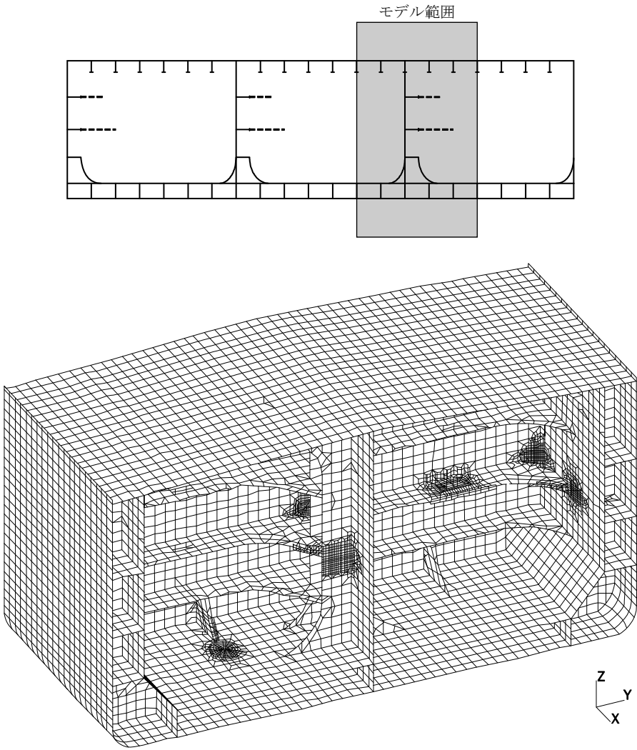
図 14 局部モデルを用いた横隔壁構造の局部解析の例
