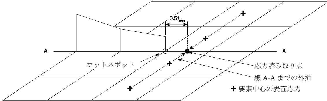
図 15 4 節点要素の応力読み取り点及びホットスポット応力の定義
