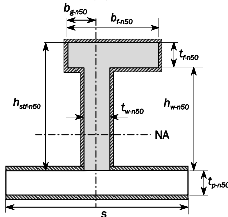
図 6 防撓材ネット寸法
