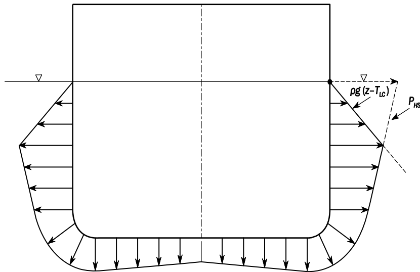
図 2 荷重ケース HSM-1, HSA-1 及び FSM-1 における船体中央での動圧の横方向分布
