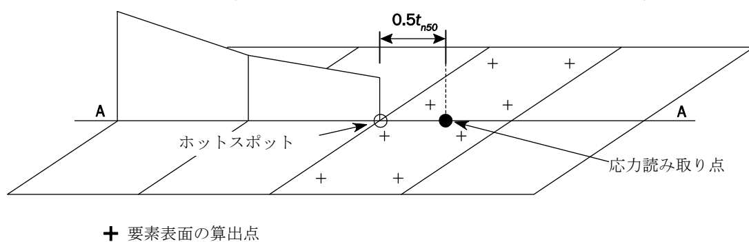
図 16 8 節点要素の応力読み取り点及びホットスポット応力の定義
