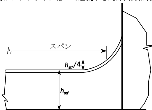
図3 面材がブラケットに沿って連続する局部支持部材の有効曲げスパン
