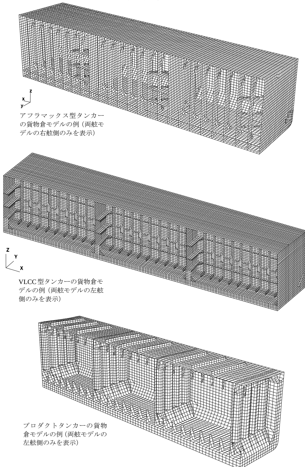
図3 油タンカーの中央部区域内における3ホールドモデルの例
