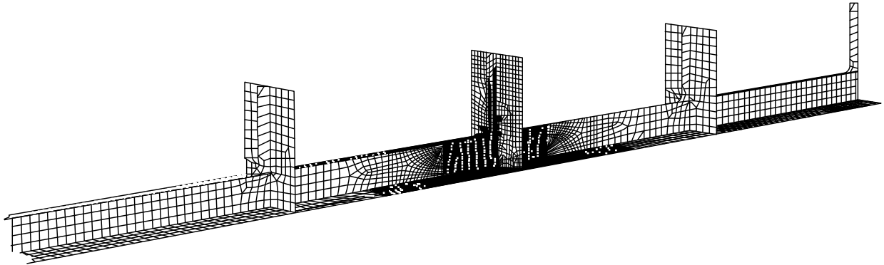
図 10 幾何学的な応力集中係数導出のための極詳細メッシュ有限要素モデル
