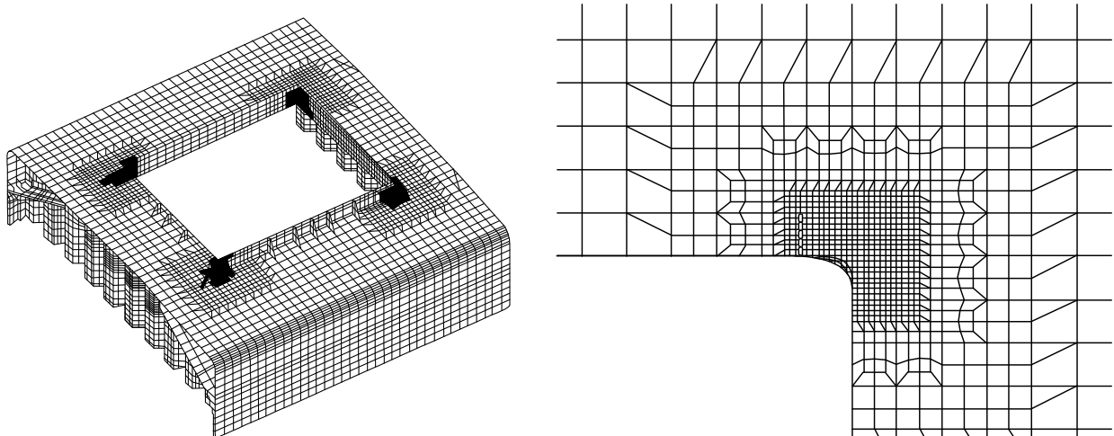
図 21 ハッチ開口部周辺構造の解析に用いる局部モデルの例
