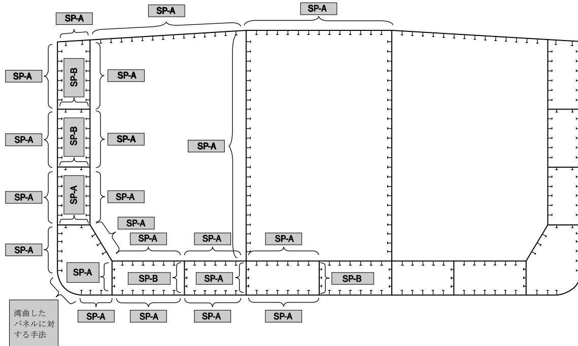
図 1 油タンカーの縦通板部材
