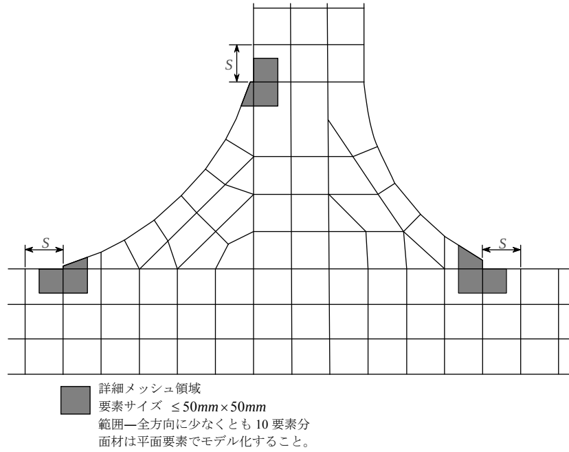
図9 ブラケット端部における詳細メッシュ領域
