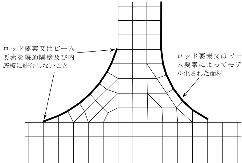
図 10 横桁の裏当てブラケットの標準的な有限要素メッシュ
