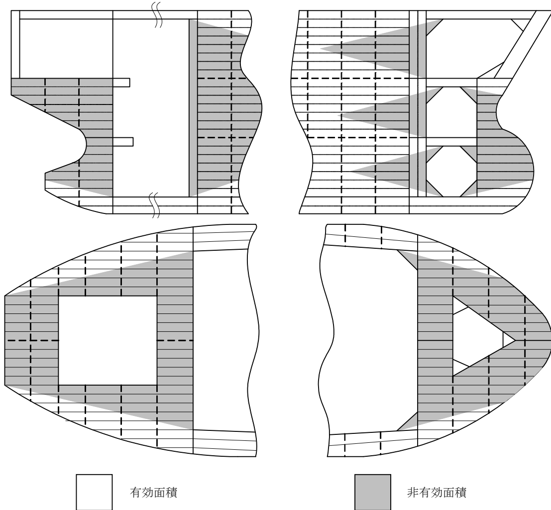
図2 不連続の甲板及び縦通隔壁の有効面積
