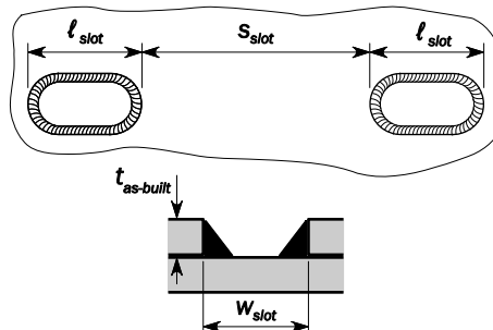
図 9 スロット溶接
