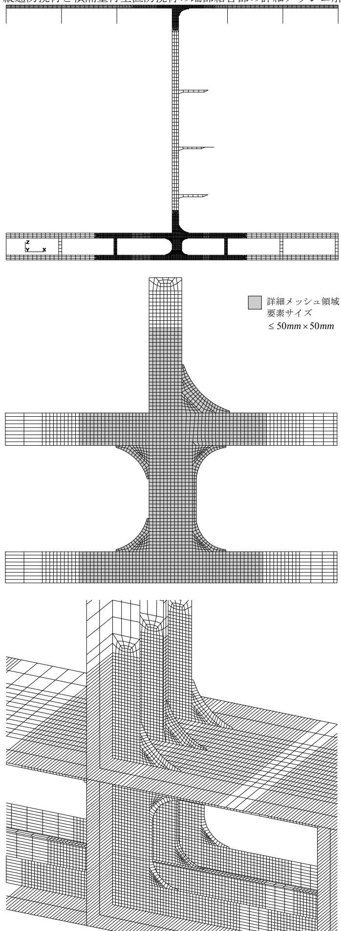
図 17 上甲板及び二重底の縦通防撓材と横隔壁付垂直防撓材の端部結合部の詳細メッシュ解析に用いる局部モデルの例
