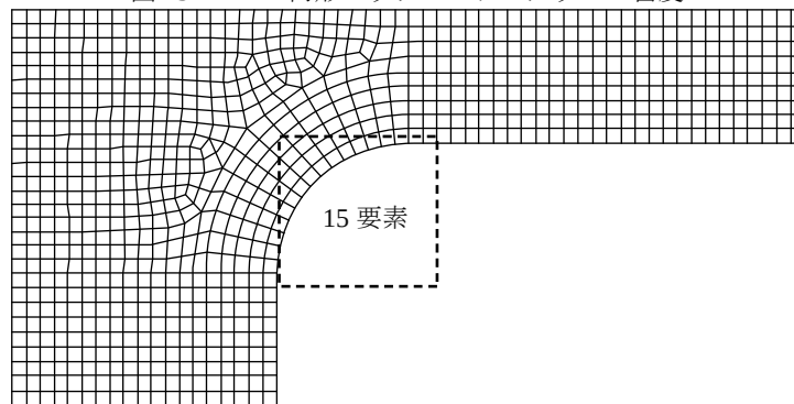
図 13 円形ハッチコーナのメッシュ密度
