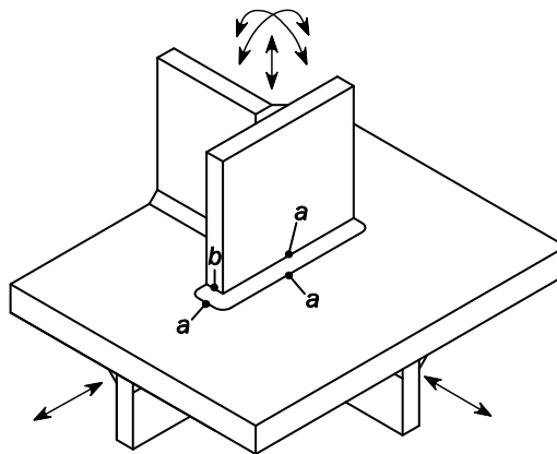
図 1 ホットスポットのタイプ
