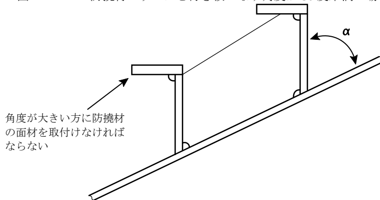
図 2 防撓材のウェブと付き板のなす角度が 50 度未満の場合
