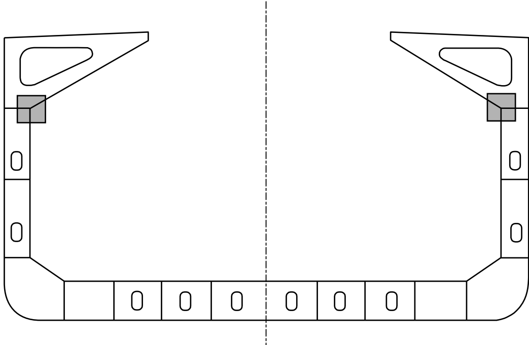
図 6 トップサイドタンクと二重船側の結合部におけるスクリーニング箇所
