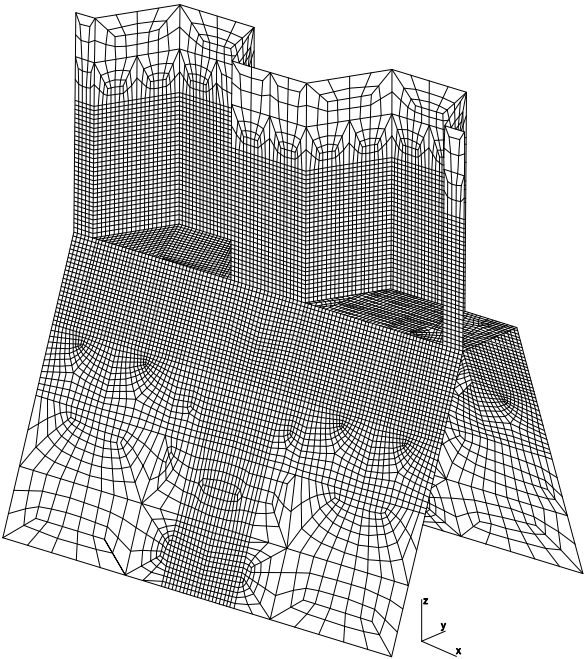
図 19 波形隔壁と下部スツールとの結合部の解析に用いる部分的な局部モデルの例
