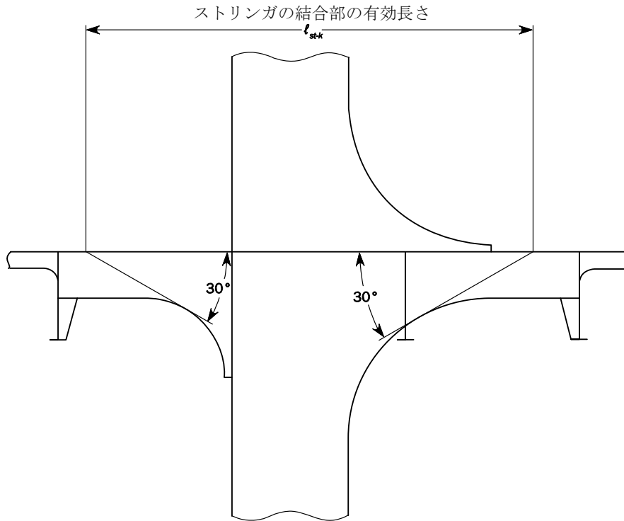
図 7 ストリングの結合部の有効長さ
