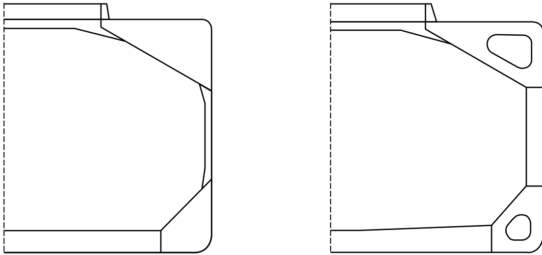
図 2 ホッパタンク及び／又はトップサイドタンクを有さない場合の貨物倉横断面の例
