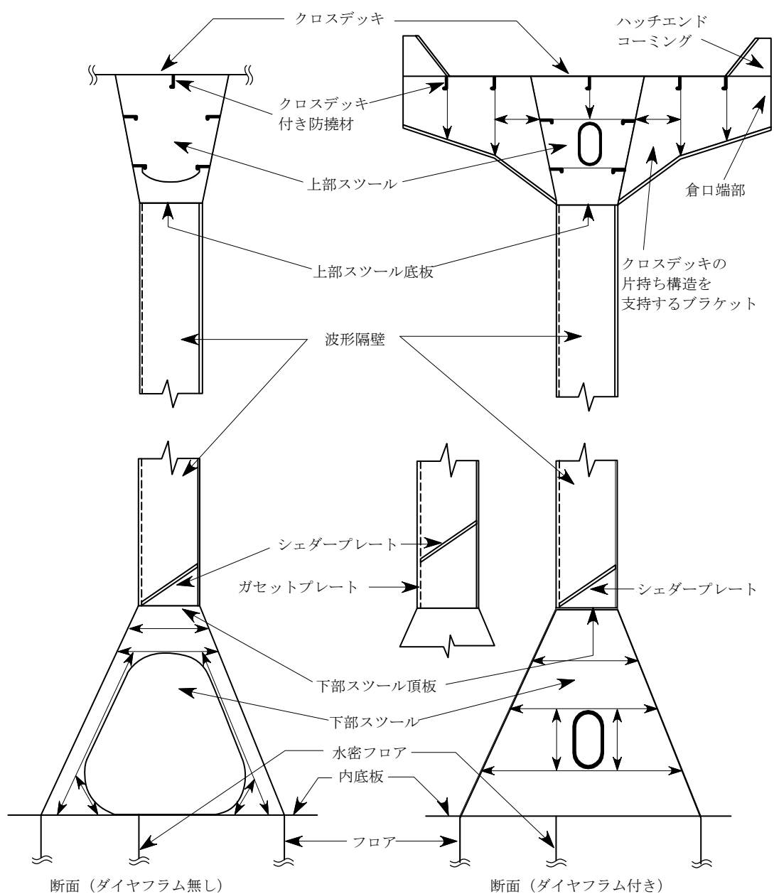
図 8 ばら積貨物船の横隔壁
