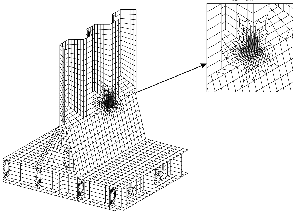
図9 波形隔壁と下部スツール板との結合部の局有限要素モデル, t_{n50} \times t_{n50} メッシュ
