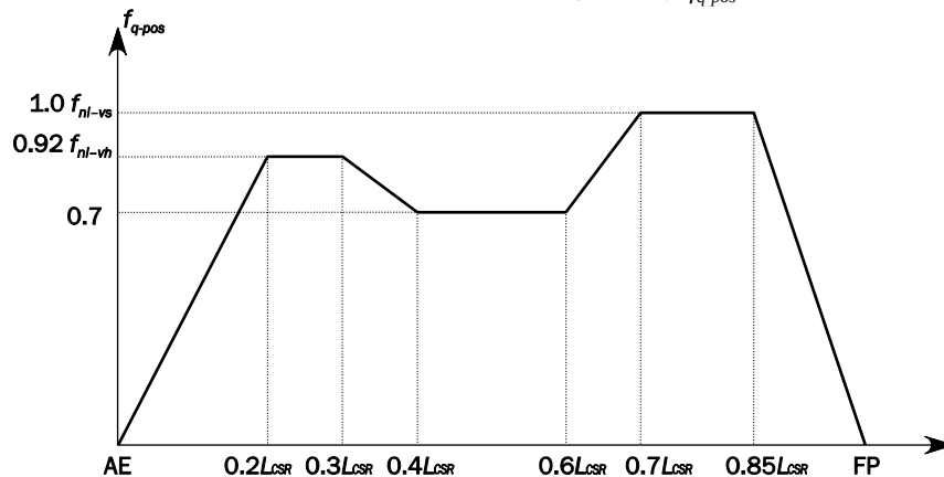
図3 正のせん断力の分布係数 f_{q-pos}
