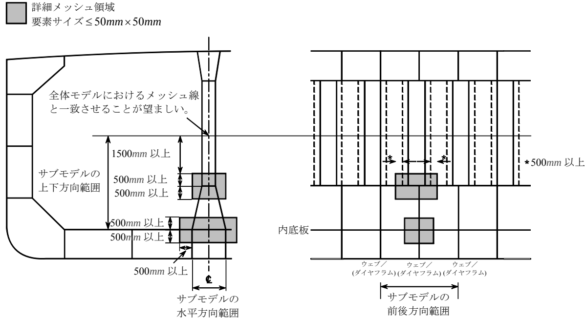
図 18 波形隔壁と下部スツールとの結合部の解析に用いる局部モデルの範囲及び詳細メッシュ領域
