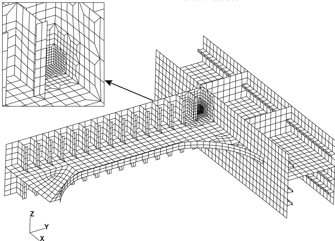
図7 スtringのヒール結合部の有限要素モデル
