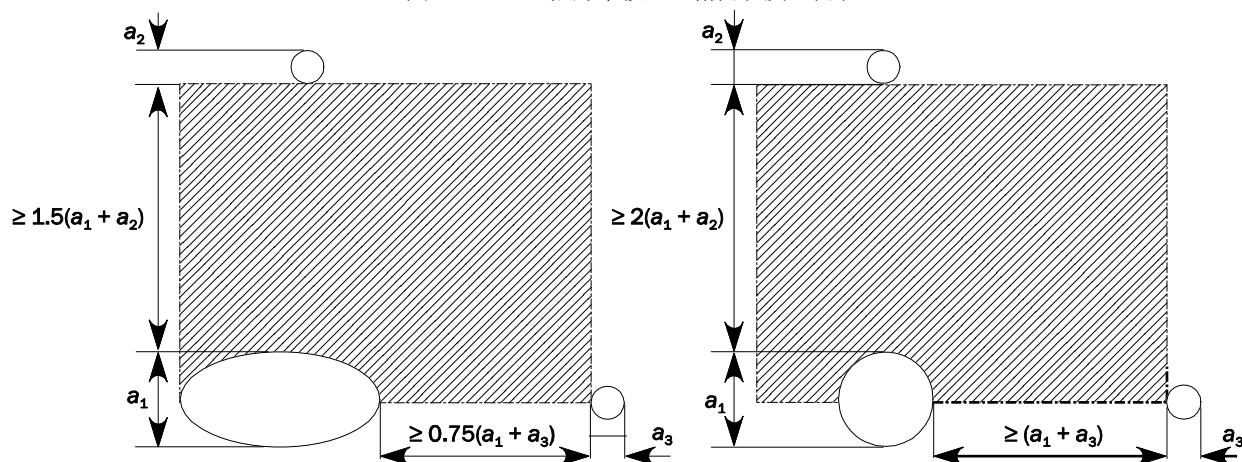
図 16 強力甲板上の楕円孔及び円孔
