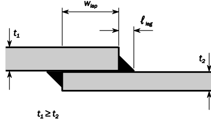
図 8 重ね継手におけるすみ肉溶接
