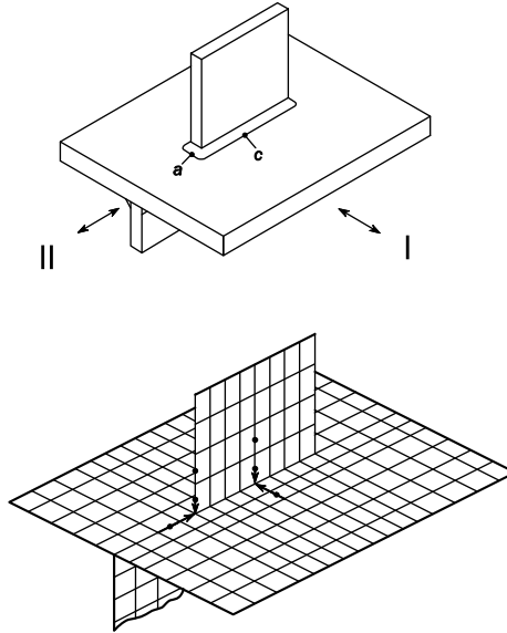
図 22 平面荷重が働く場合の垂直溶接付加物の評価箇所
