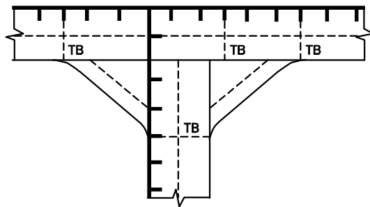
端部ブラケット先端部のトリッピングブラケット
