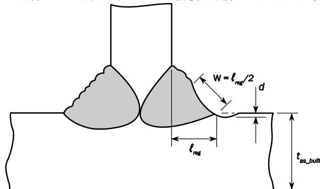
図 6 内部ビードを除去するための溶接止端部のグラインディングの範囲
