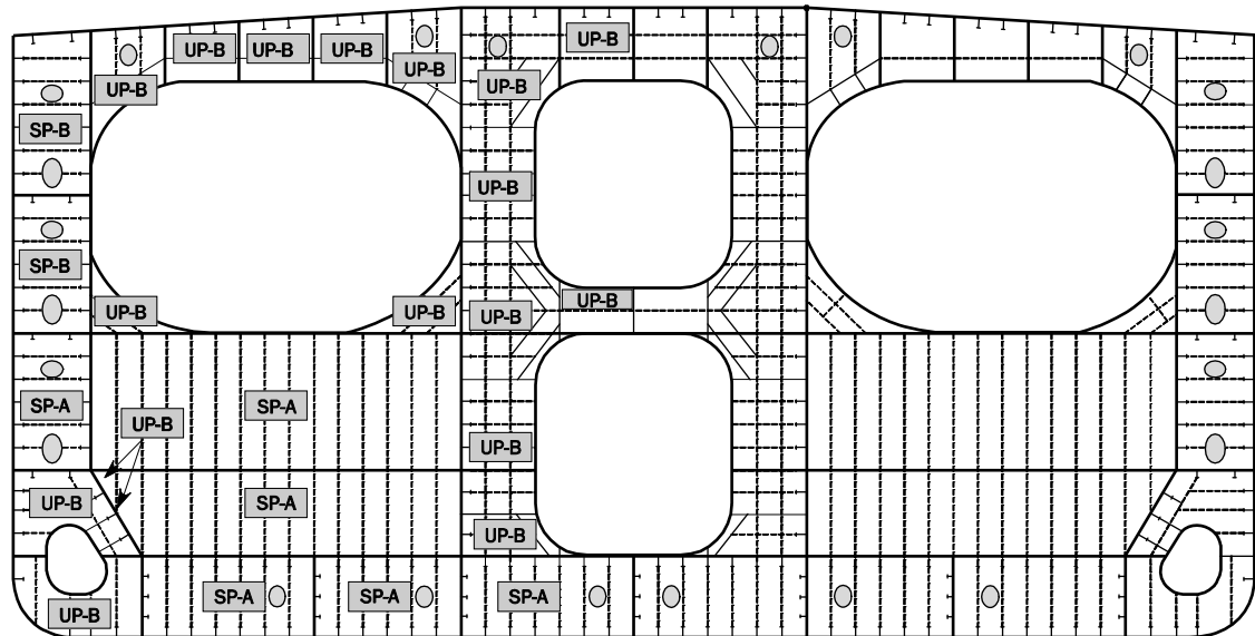
図4 クロスタイ
