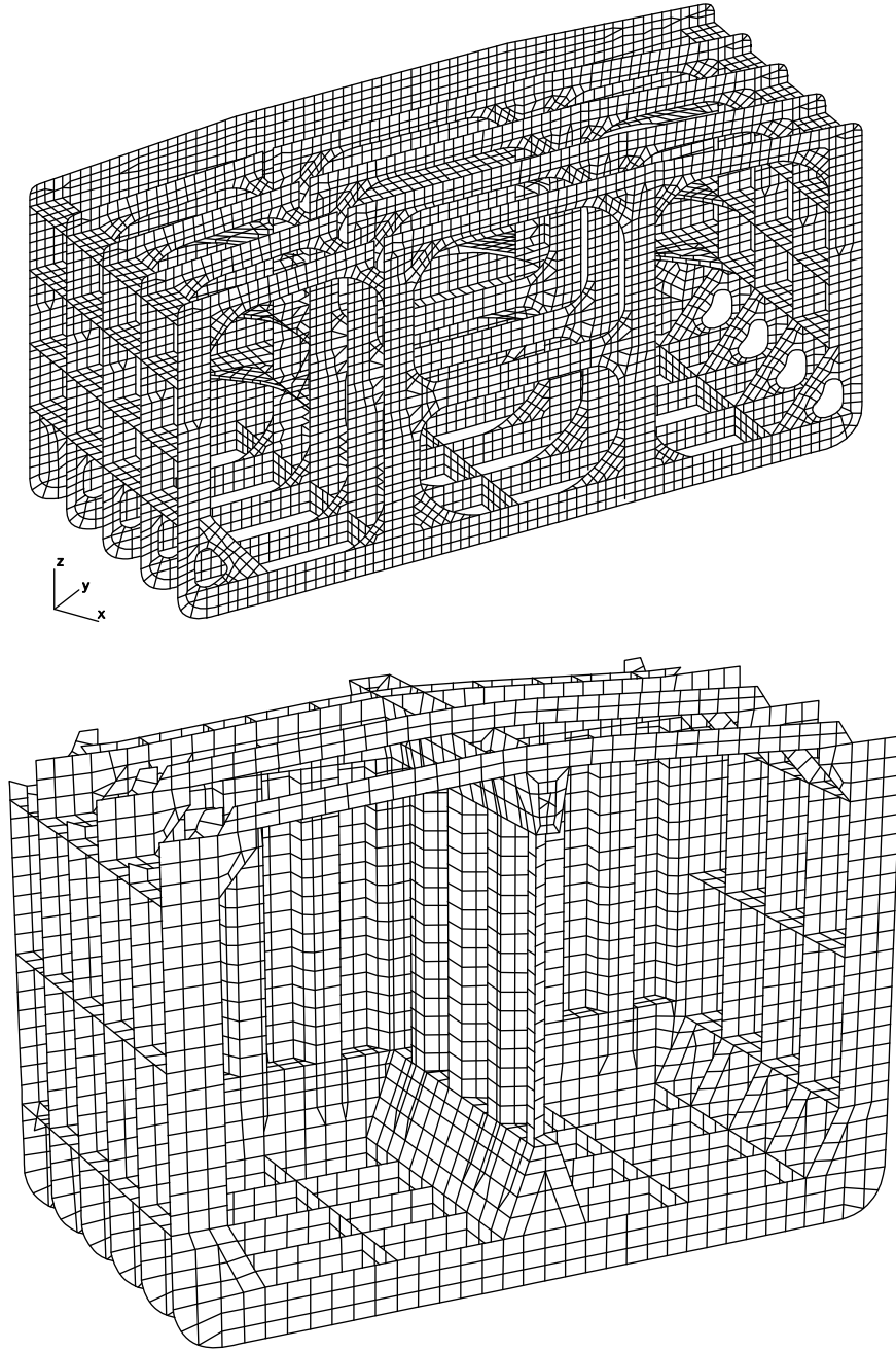
図 14 VLCC 型タンカー及びプロダクトタンカーの貨物タンク構造の有限要素メッシュ配置の例
