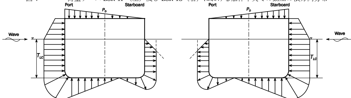
図 4 荷重ケース BSR-1P (左) 及び BSR-1S (右) における船体中央での動圧の横方向分布
