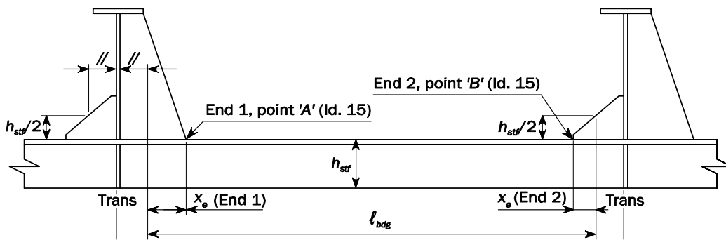
横方向の自由端フランジによる支持
