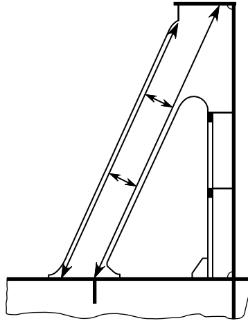
図 4 ハッチコーミングステイ (例 3)
