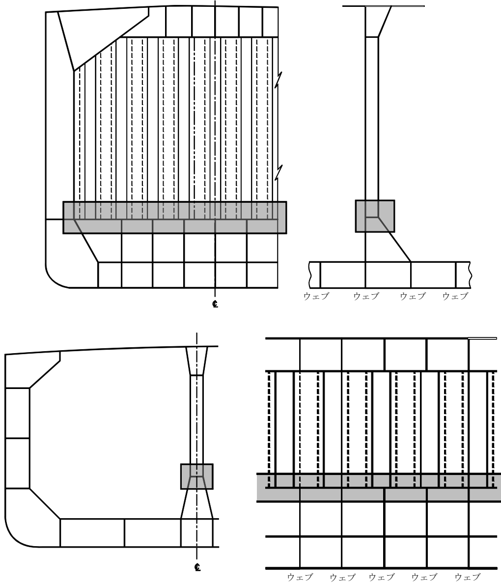
図4 波形隔壁と下部スツールとの結合部における評価必須箇所
