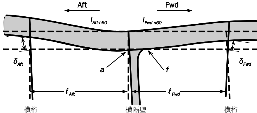
図 4 相対変位の定義 (船側縦通防撓材の例)
