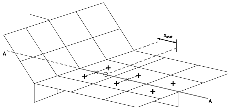
図 20 桁等で支持された十字継手の応力読み取り点の求め方
