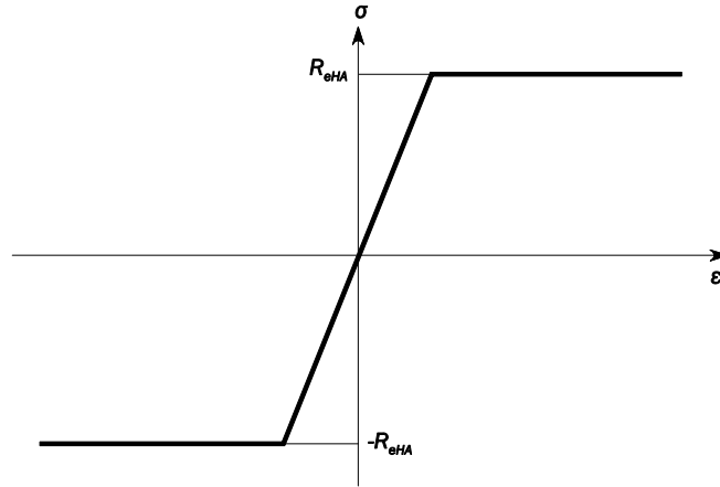
図7 弾塑性崩壊に対する応力-ひずみ曲線 \sigma-\varepsilon
