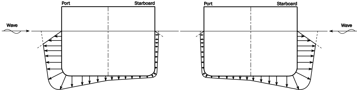
図 11 荷重ケース OSA-2P (左) 及び OSA-2S (右) における船体中央での動圧の横方向分布
