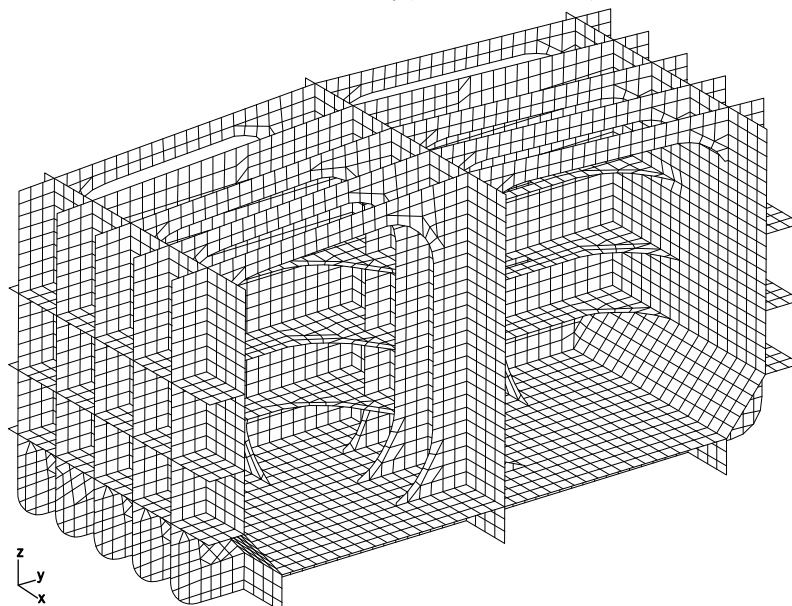
図 13 アフラマックス型タンカーの貨物タンク構造の有限要素メッシュ配置の例
