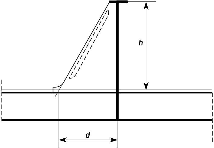
図 3 トリップングブラケットの有効長さ
