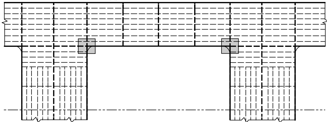
図8 ばら積貨物船のハッチコーナにおけるスクリーニング箇所
