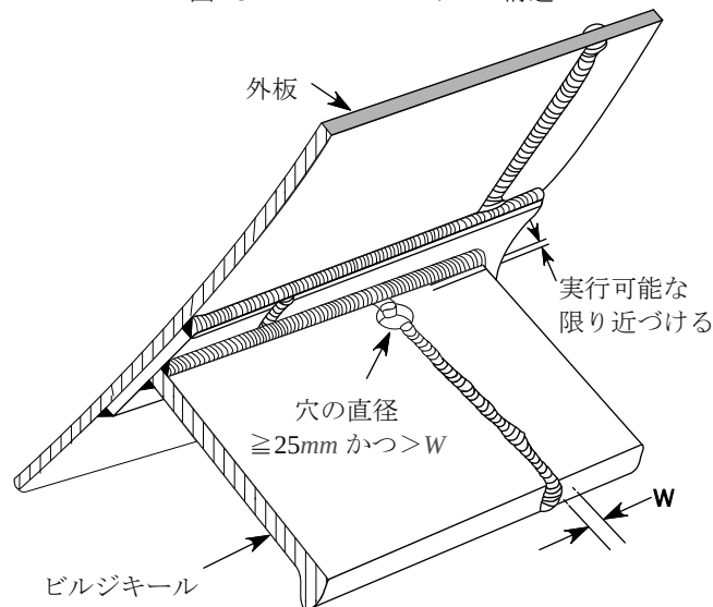
図 18 ビルジキール構造
