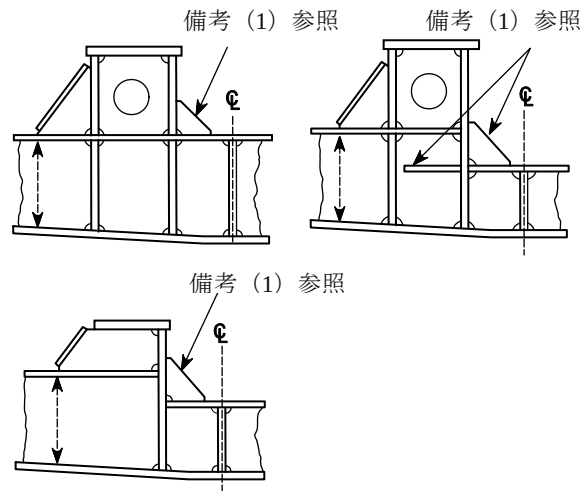
図2 機器の台座 タイプ2
