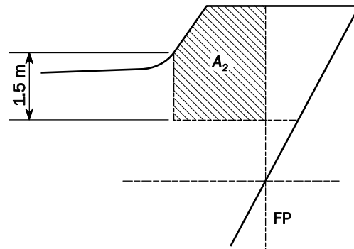
図 2 スクリーン及びブルワークの側面積
