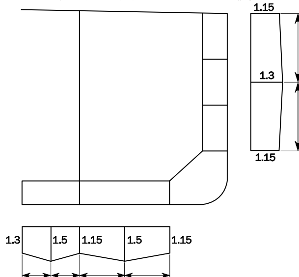
図3 2列の縦通隔壁を有する油タンカーの満載状態における係数 K_d
