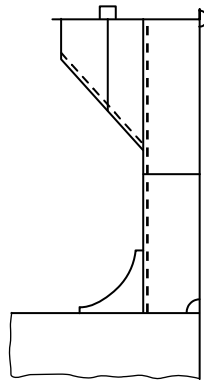
図 3 ハッチコーミングステイ (例 2)
