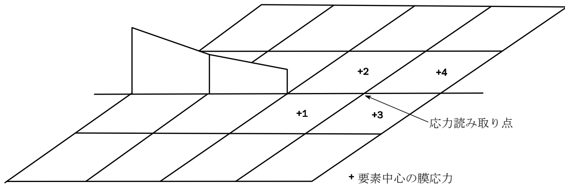
図 23 ブラケット先端部における応力読み取り点
