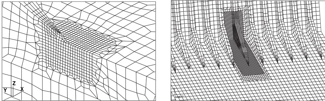
図10 開口部周りの詳細メッシュ領域
