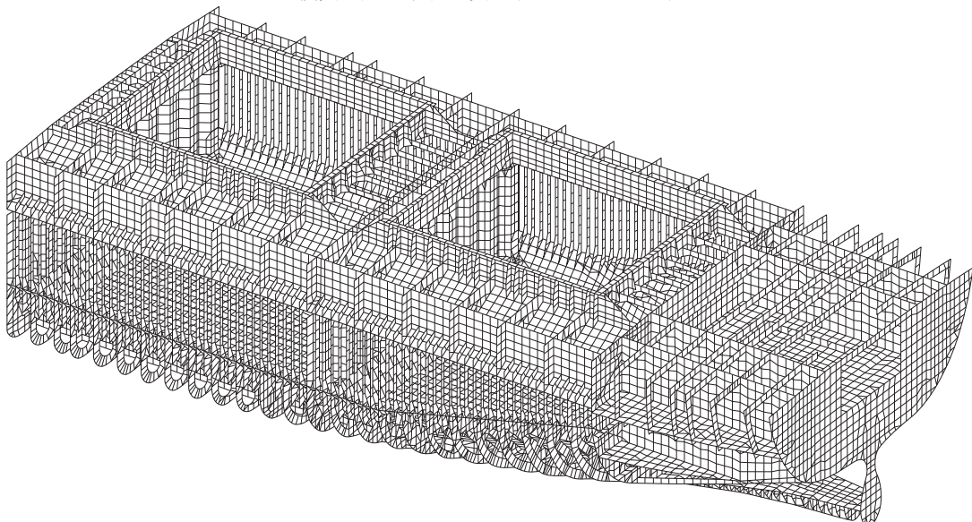
図 6 ばら積貨物船の最後端貨物倉構造に対する有限要素モデルの例
