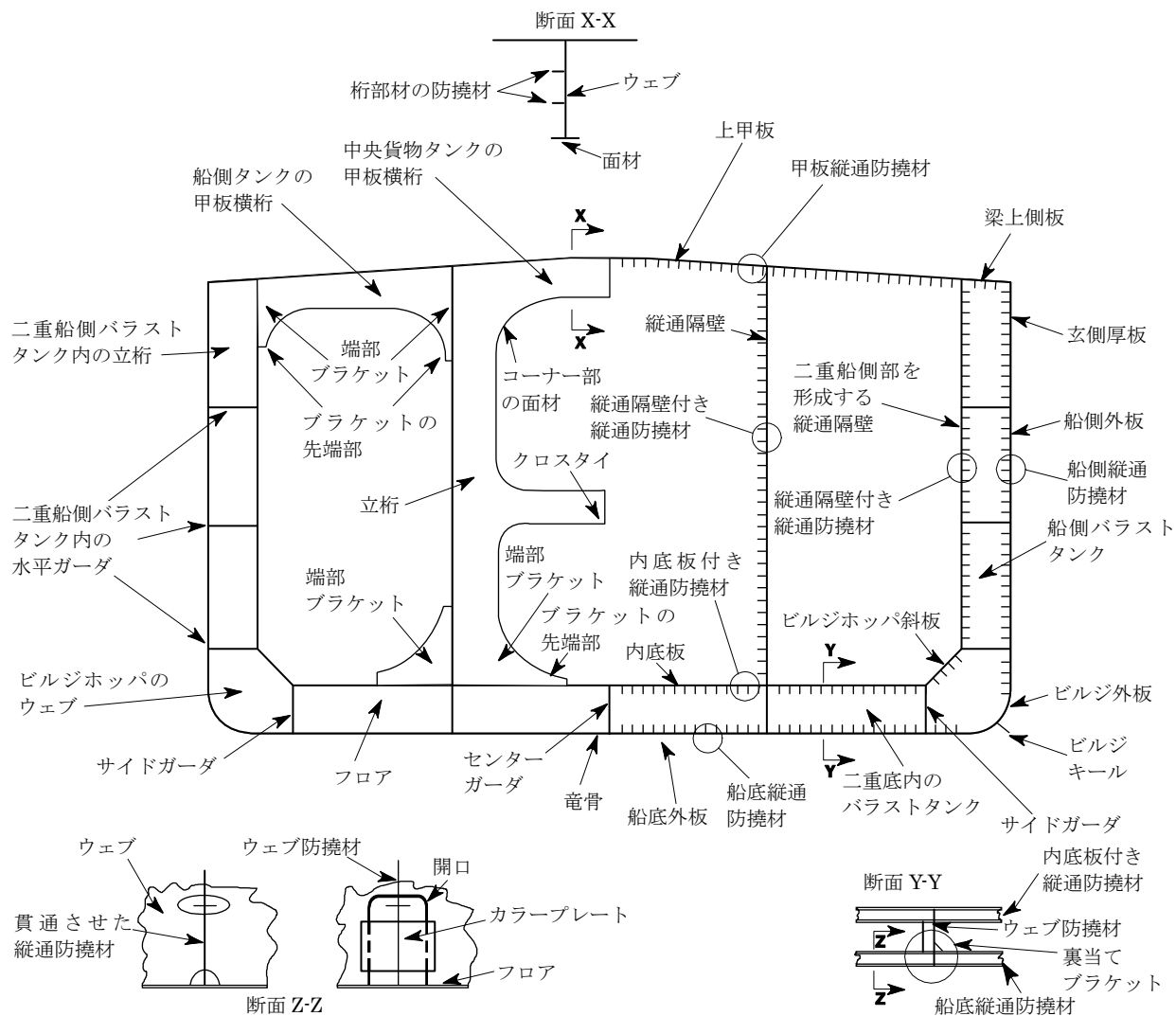
図6 二重船殻タンカーの中央部貨物タンクの横断面
