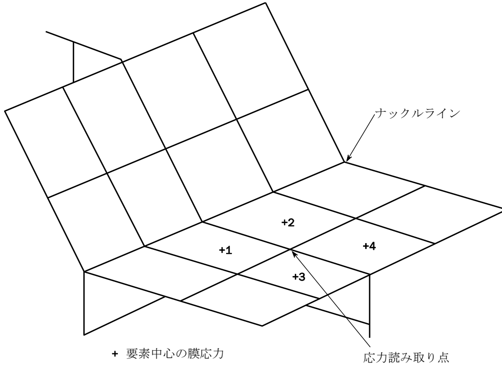
図 24 ナックル部の詳細の応力読み取り点
