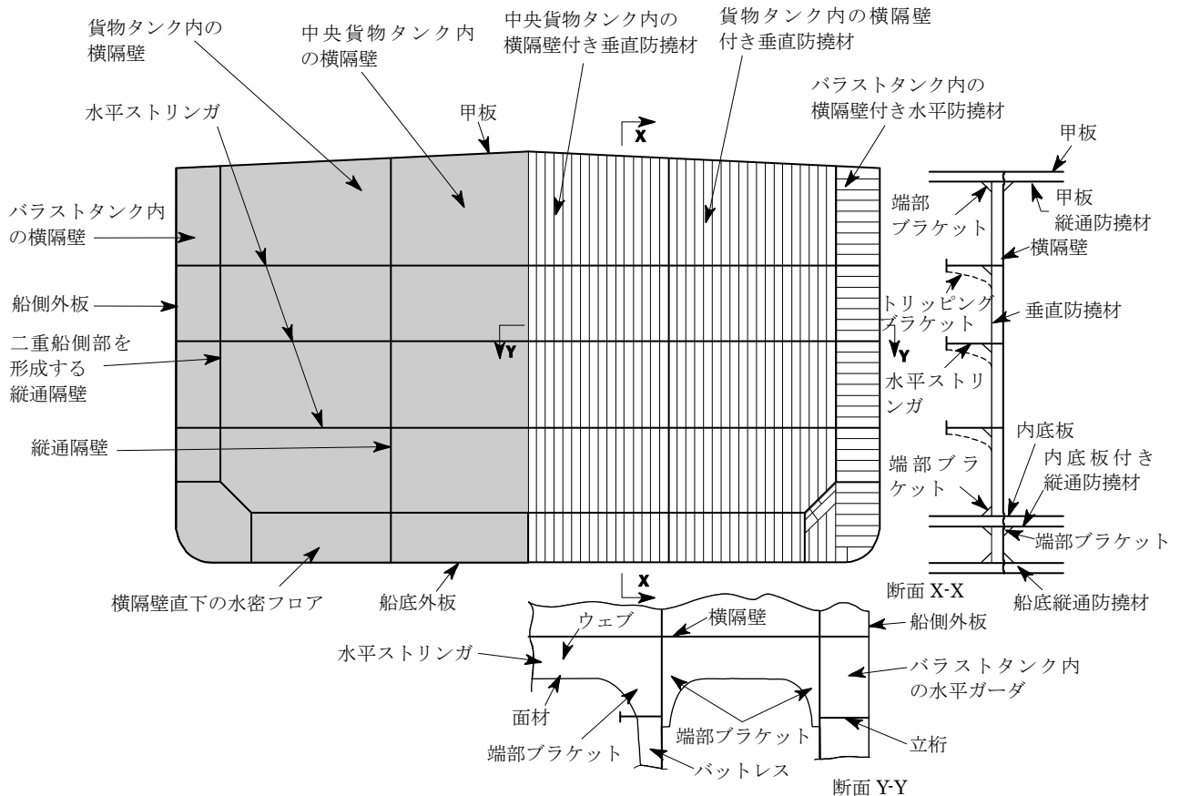
図 5 二重船殻タンカーの横隔壁
