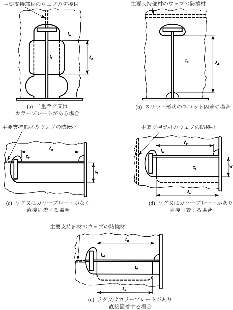
図 8 対称形状及び非対称形状のスロット
