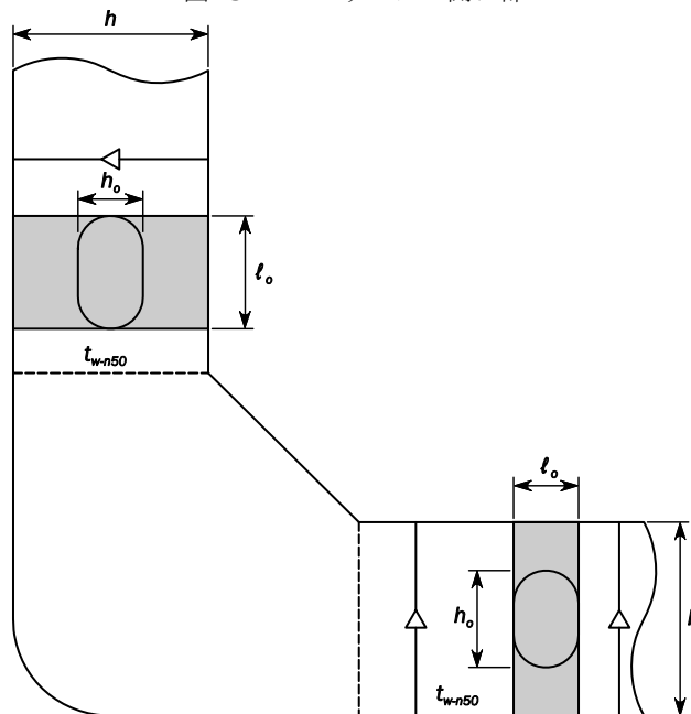
図 15 ウェブの開口部
