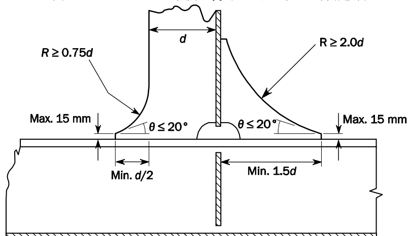
梁柱防撓材のソフトトウ及び裏当てブラケットの推奨設計
