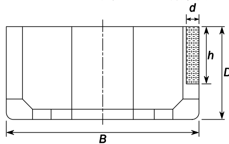
図 1 衝突による損傷範囲
