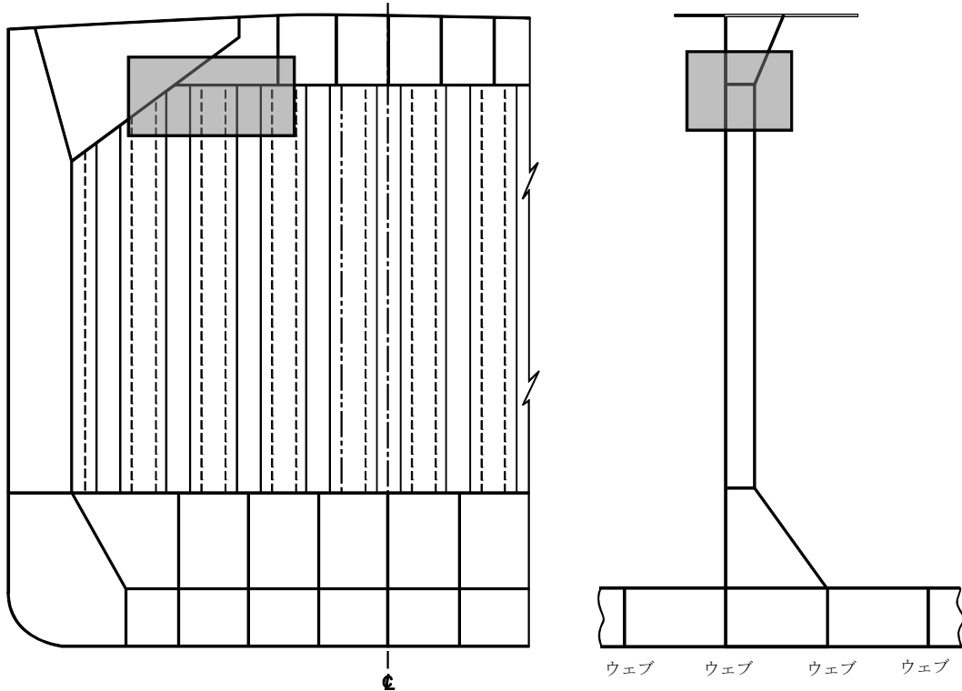
図7 波形隔壁と上部スツールを含む上部支持構造との結合部におけるスクリーニング箇所
