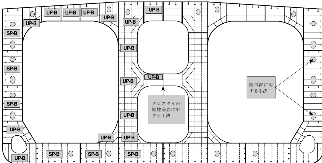
図2 油タンカーの横部材
