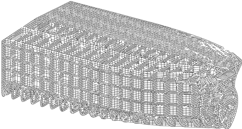
図 5 油タンカーの最前端貨物倉構造に対する有限要素モデルの例
