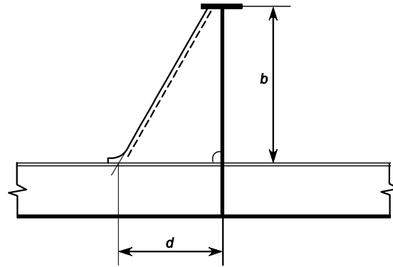
防撓材近傍のトリッピングブラケット
