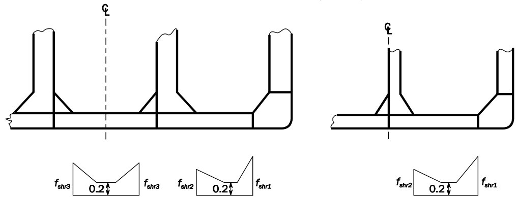
図 1 フロアのせん断力分布係数
