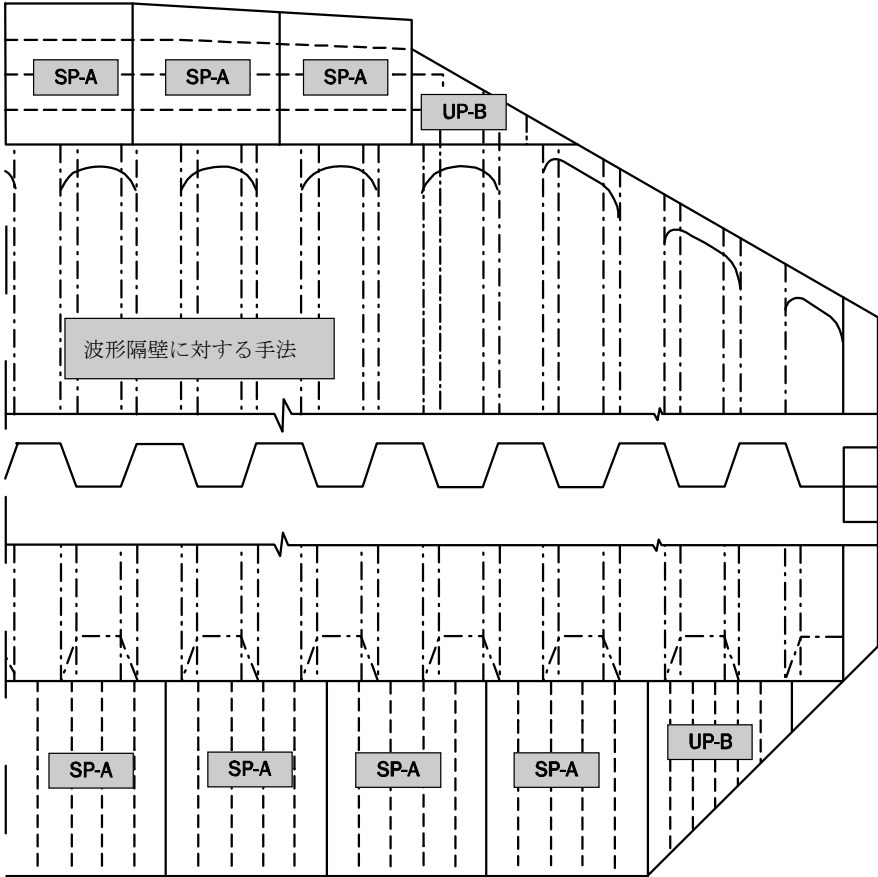
図 9 ばら積貨物船の波形隔壁及びクロスデッキ
