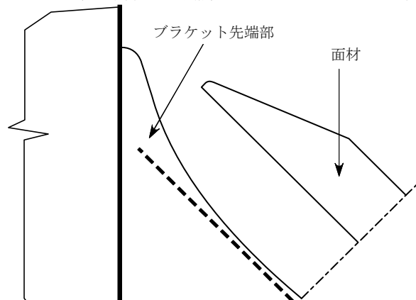
図6 遊縁に隣接した箇所に設けるブラケットの面材
