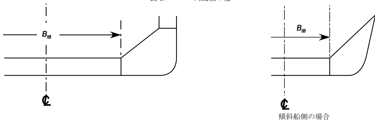
図 17 内底板の幅
