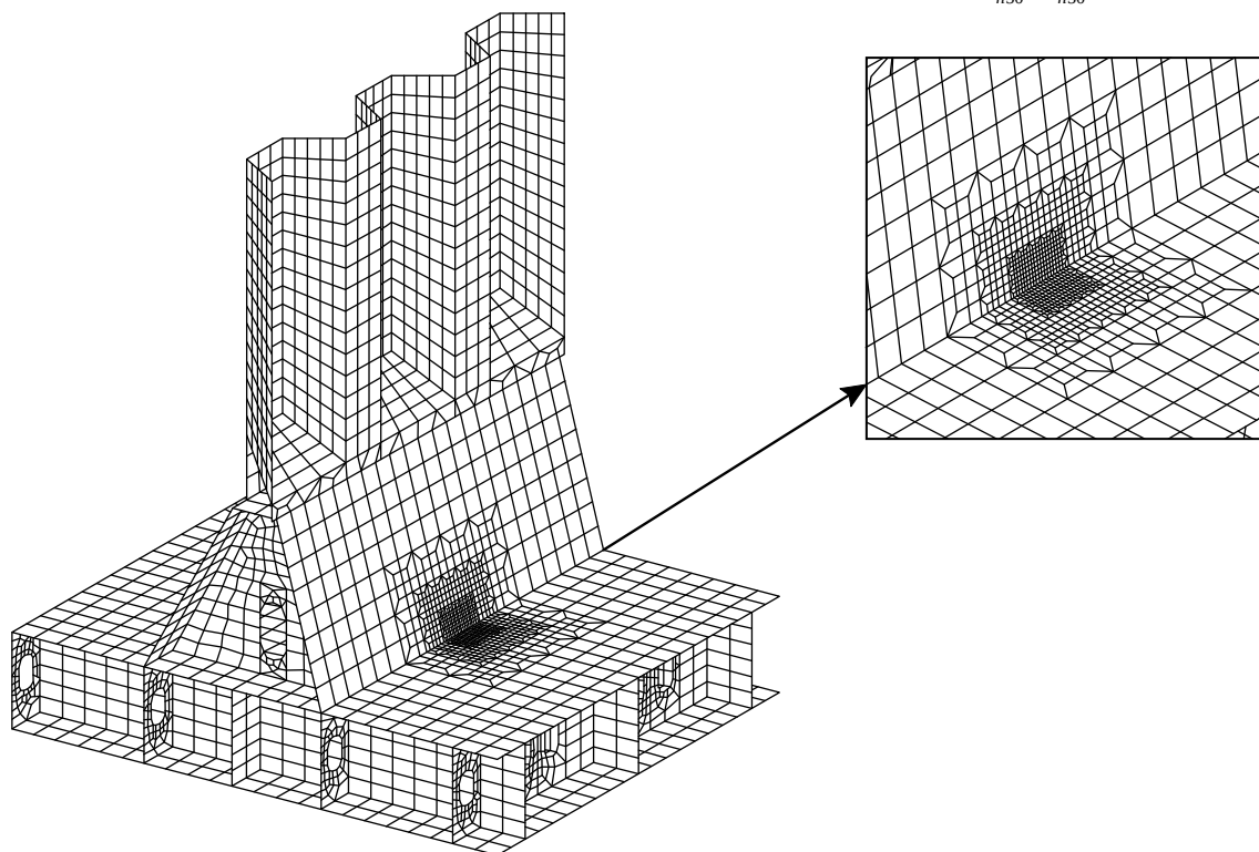
図8 内底板と下部スツール斜板との結合部の局有限要素モデル, t_{n50} \times t_{n50} メッシュ
