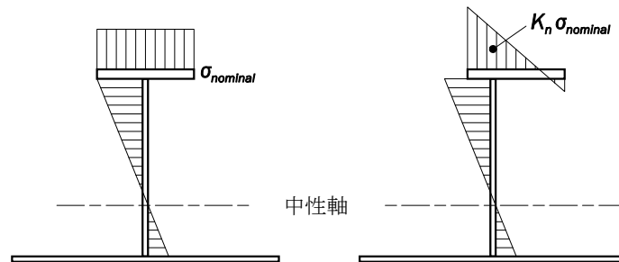
図 5 対称及び非対称フランジを持つ防撓材の曲げ応力
