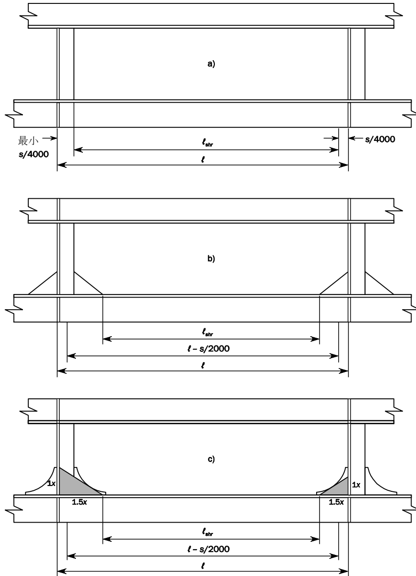
図 5 ウェブ防撓材に支持される防撓材の有効せん断スパン（二重船殻構造）
