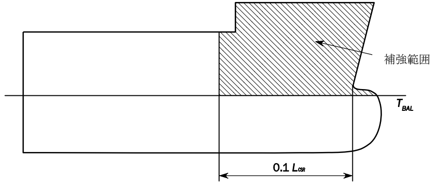
図 4 船首衝撃に対する補強範囲
