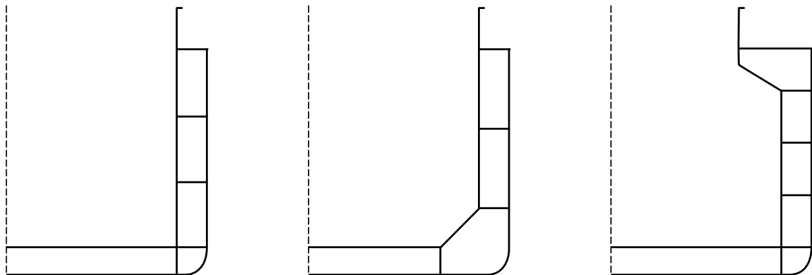
図 2 ホッパタンク及び／又はトップサイドタンクを有さない場合の貨物倉横断面の例
