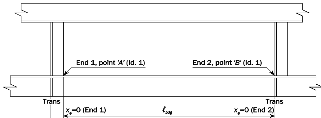
二重船側/横隔壁による支持
