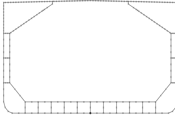
図 18 ばら積貨物船の端部ビーム要素
