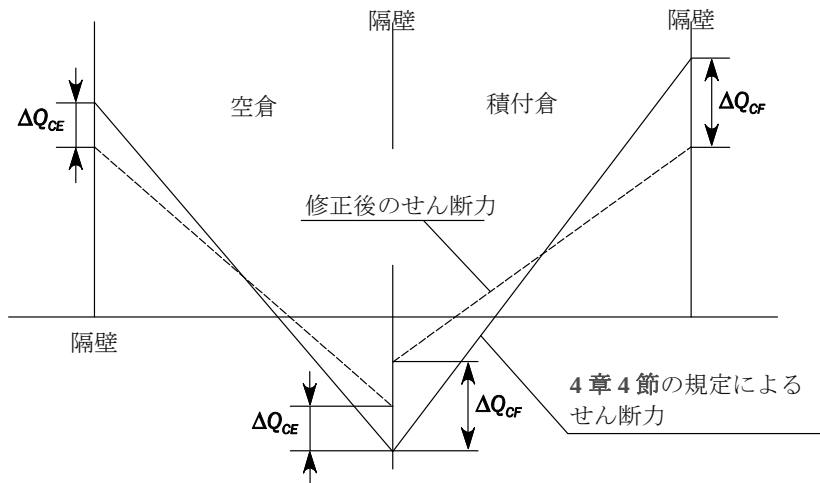
図 11 せん断力修正 \Delta Q_C
