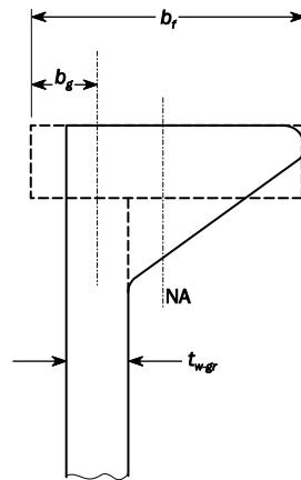
図 7 バルブプレート及び等価な組立形鋼
