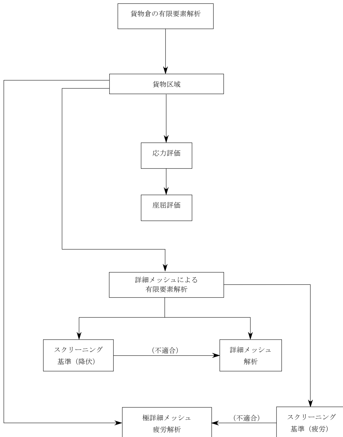
図 1 有限要素解析のフロー図
