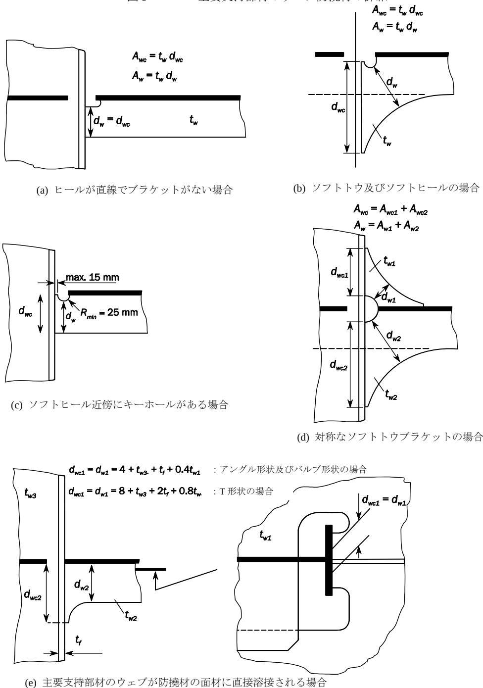
図 9 主要支持部材のウェブ防撓材の詳細
