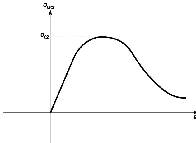
図 9 捩れ座屈に対する応力-ひずみ曲線 \sigma_{CR2} - \varepsilon
