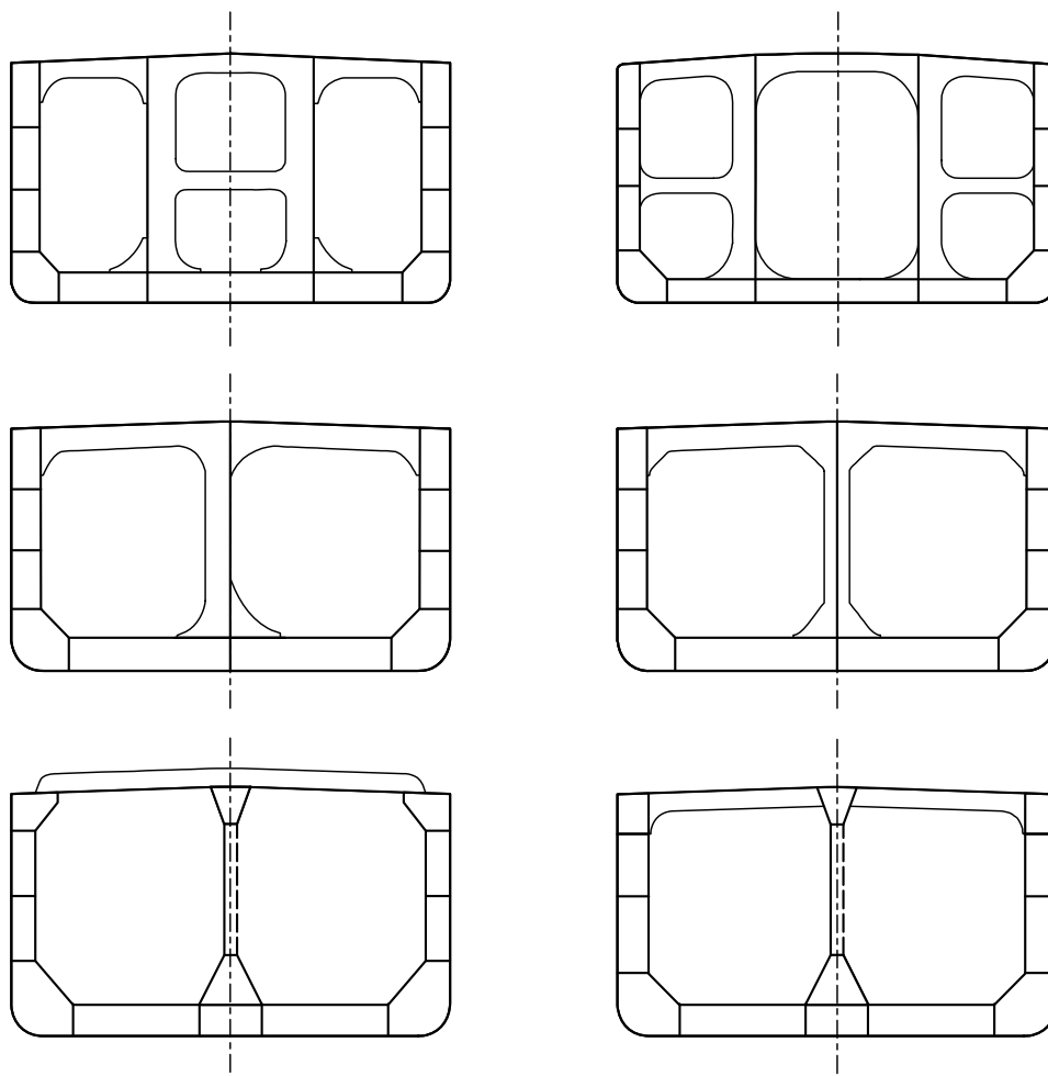
図3 二重船殻油タンカーの典型的な構造配置
