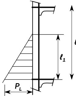
図 25 垂直防撓材に作用する面外圧力の定義
