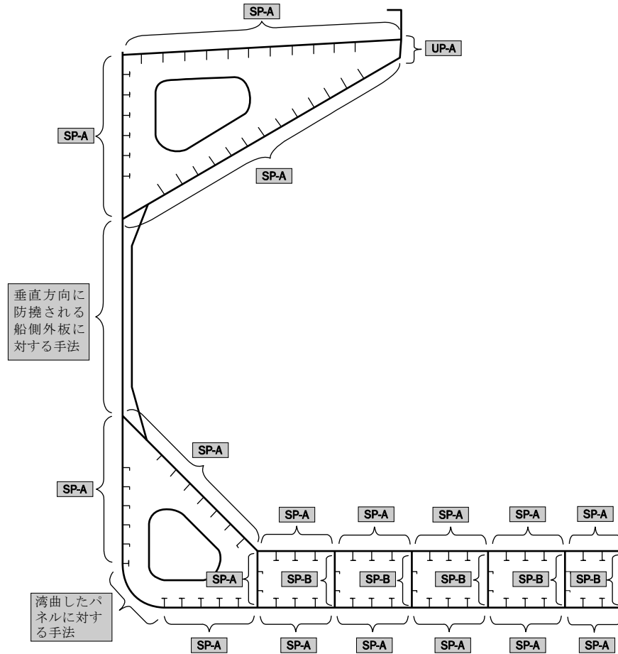
図5 単船側ばら積貨物船の縦通板部材
