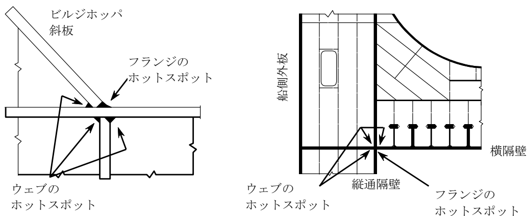
図17 桁等に支持された十字継手
