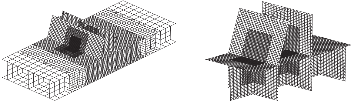
図 20 下部スツールと内底板との結合部の解析に用いる部分的な局部モデルの例
