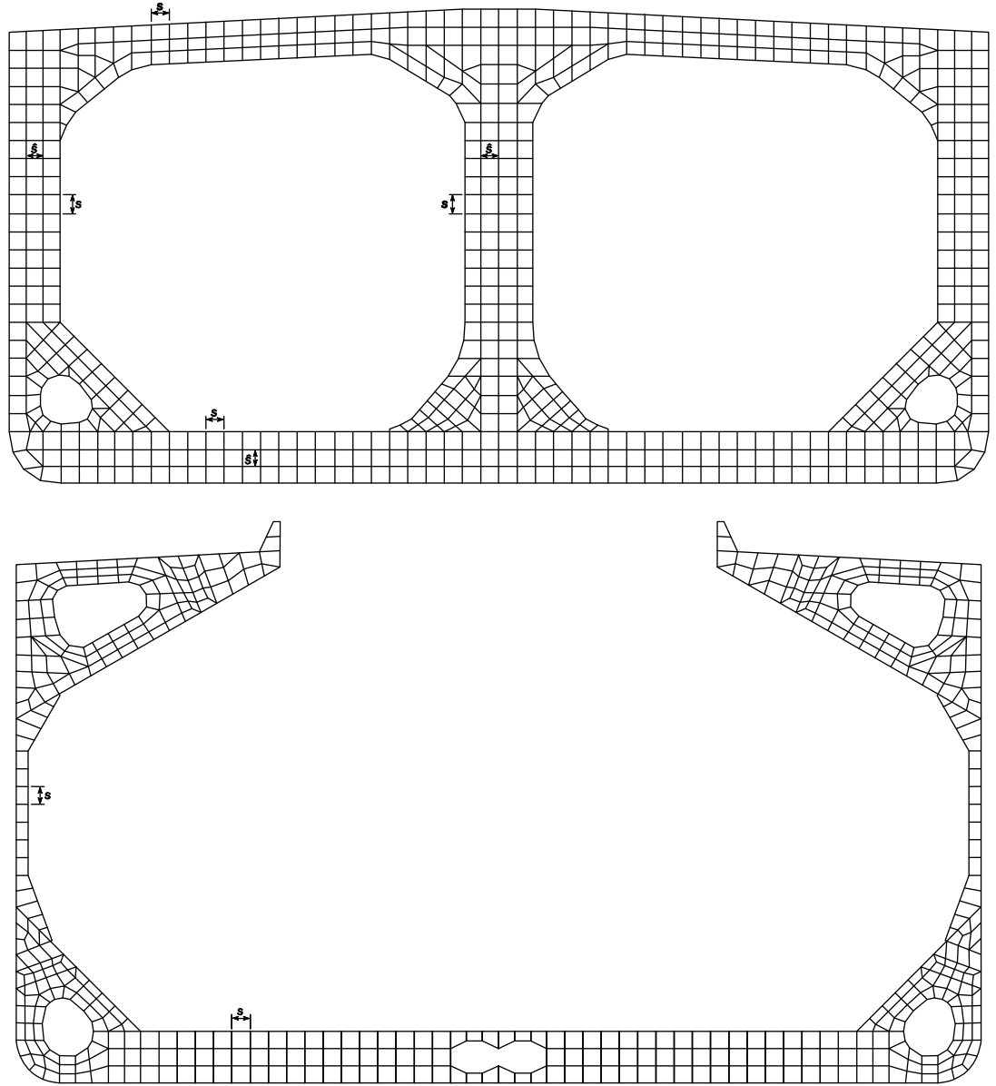
図 7 横桁の標準的な有限要素メッシュ
