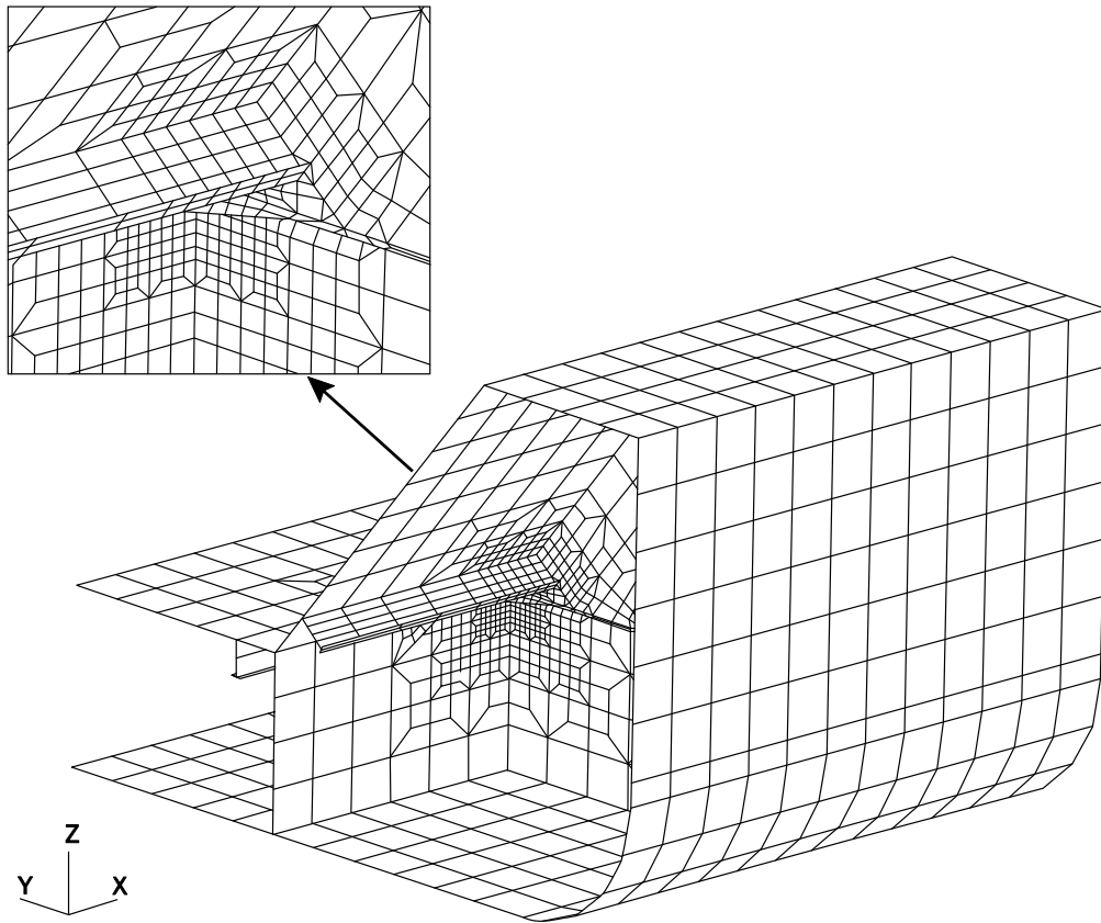
図4 内底板，ビルジホップ斜板，ウェブフレーム，ガーダ及びブラケット間のナックル結合部の局部極詳細メッシュモデル( t_{n50} \times t_{n50} )
