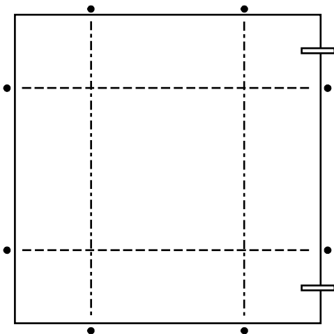
呼び寸法 1330×1330
