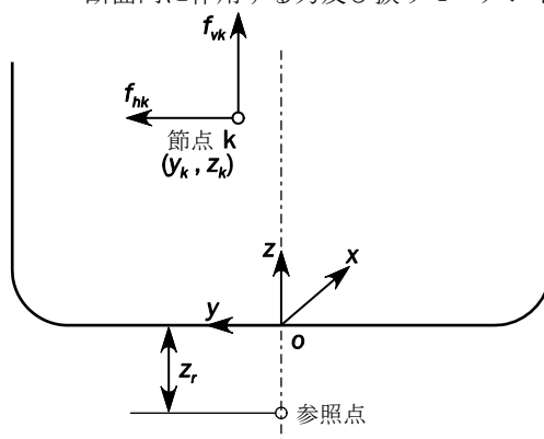
図 20 断面内に作用する力及び振りモーメントの位置
