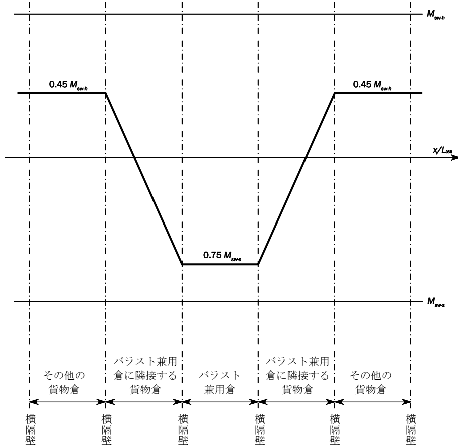
図 1 疲労強度評価のためのバラスト兼用倉の静水中縦曲げモーメントの分布
