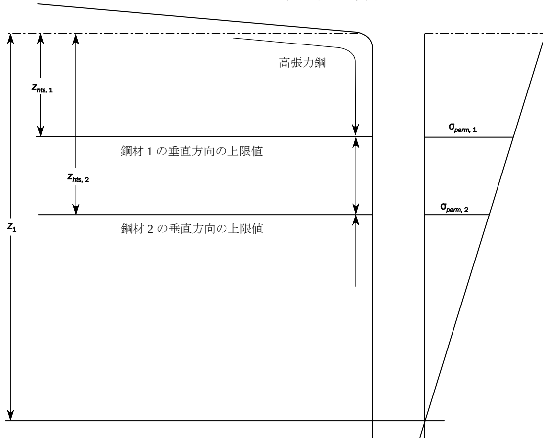
図3 高張力鋼の垂直方向範囲
