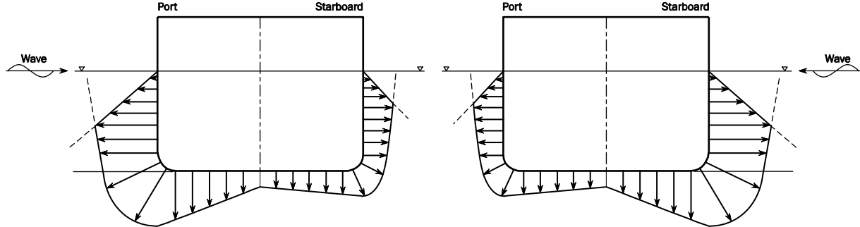
図7 荷重ケース BSP-2P (左) 及び BSP-2S (右) における船体中央での動圧の横方向分布
