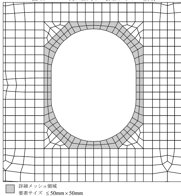
図10 開口部周りの詳細メッシュ領域
