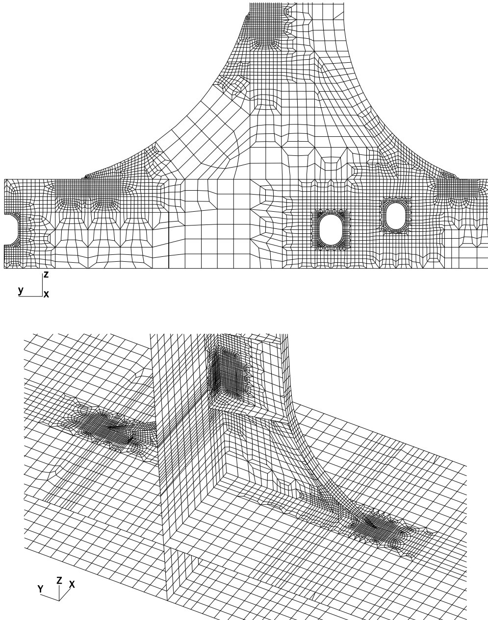
図 12 横桁下部における有限要素メッシュの拡大図
