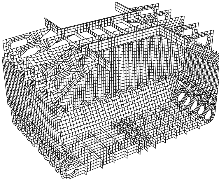
図 11 ばら積貨物船の貨物倉構造の有限要素メッシュ配置の例
