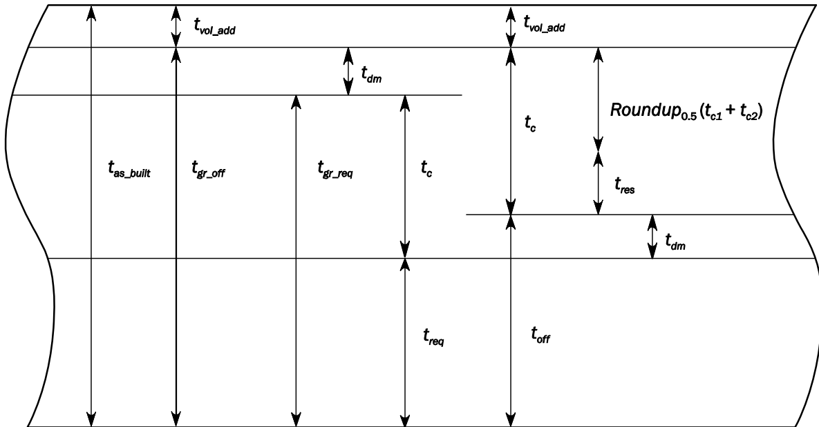
図 1 ネット寸法手法のスキーム
