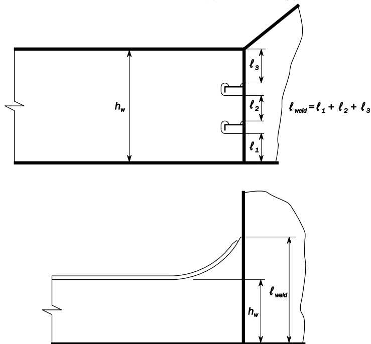
図 6 主要支持部材のせん断面積
