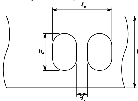
図 16 d_o < h/4 の連続した開口部に対する長さ
