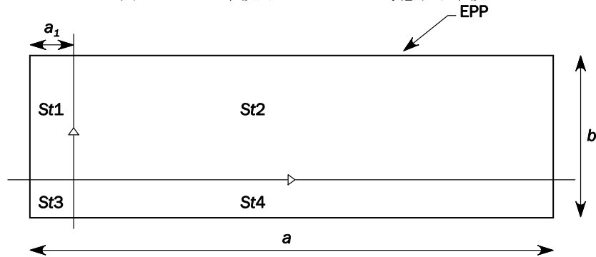
図 18 条板内の EPP として考慮する条板
