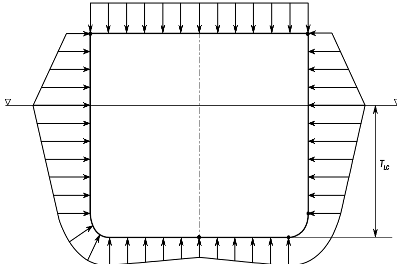
図 3 荷重ケース HSM-2, HSA-2 及び FSM-2 における船体中央での動圧の横方向分布
