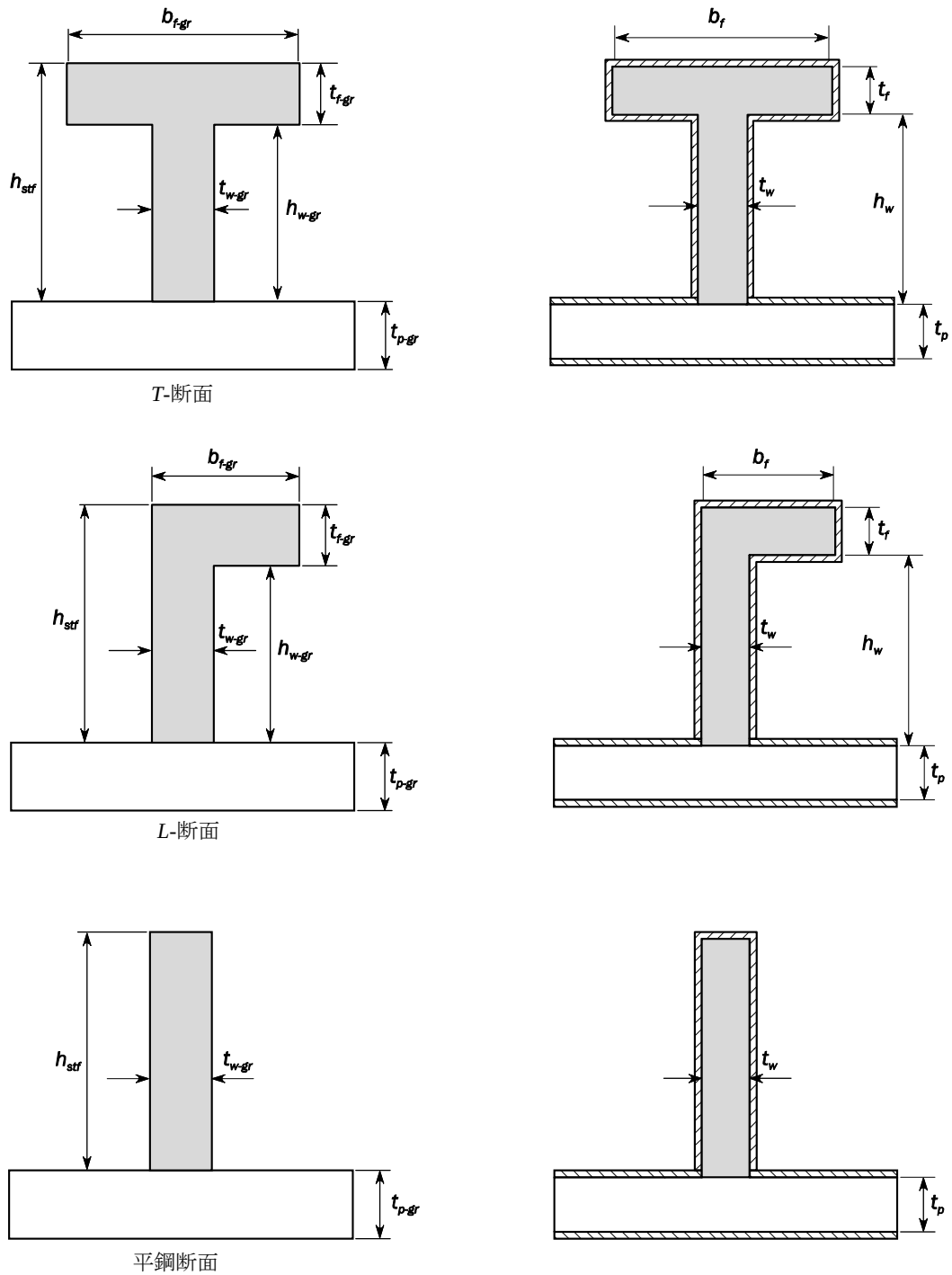
図 2 局所支持部材のネット断面特性
