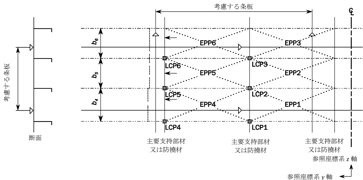
図 21 水平防撓構造の立て横部材における荷重計算点
