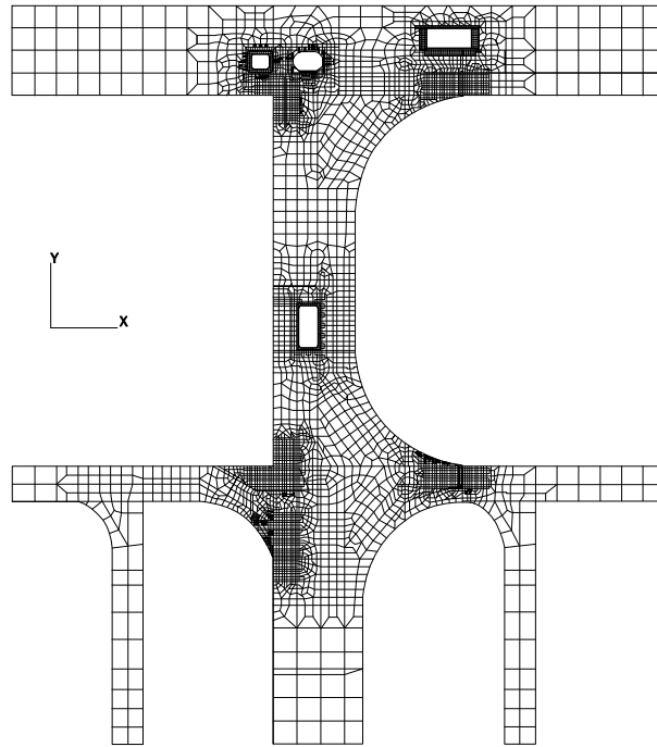
図 15 横隔壁付ストリングの有限要素メッシュ図の例
