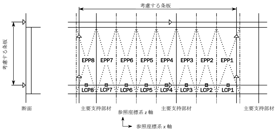
図 20 横式構造における荷重計算点 (LCP)
