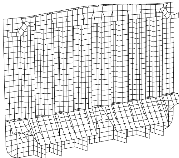
図 12 プロダクトタンカーの波形横隔壁構造の有限要素メッシュの例
