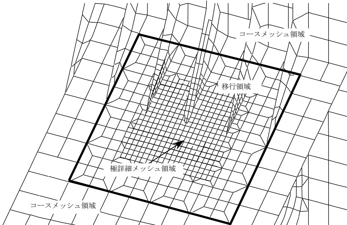
図6 コースメッシュと極詳細メッシュの移行領域
