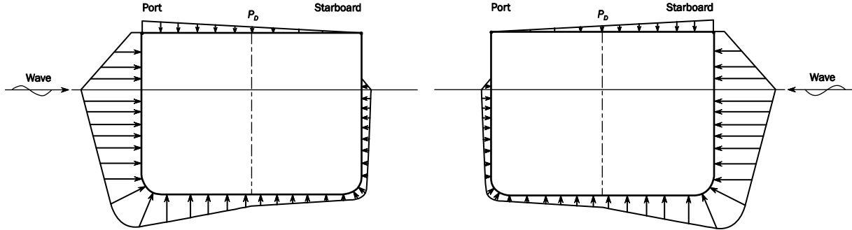
図 10 荷重ケース OSA-1P (左) 及び OSA-1S (右) における船体中央での動圧の横方向分布
