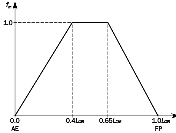
図2 分布係数 f_m
