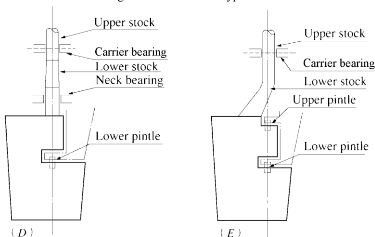
Fig. 4.2.1.1-1 Mariner-type Rudders
