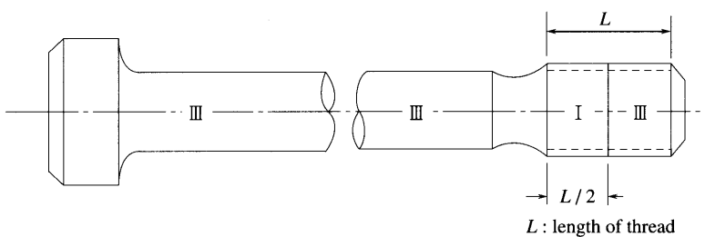
(f) Bolt
