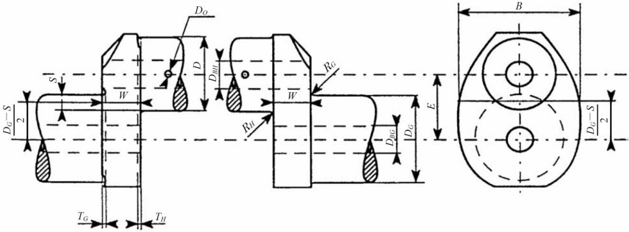
Fig. 5 Crank Dimensions
