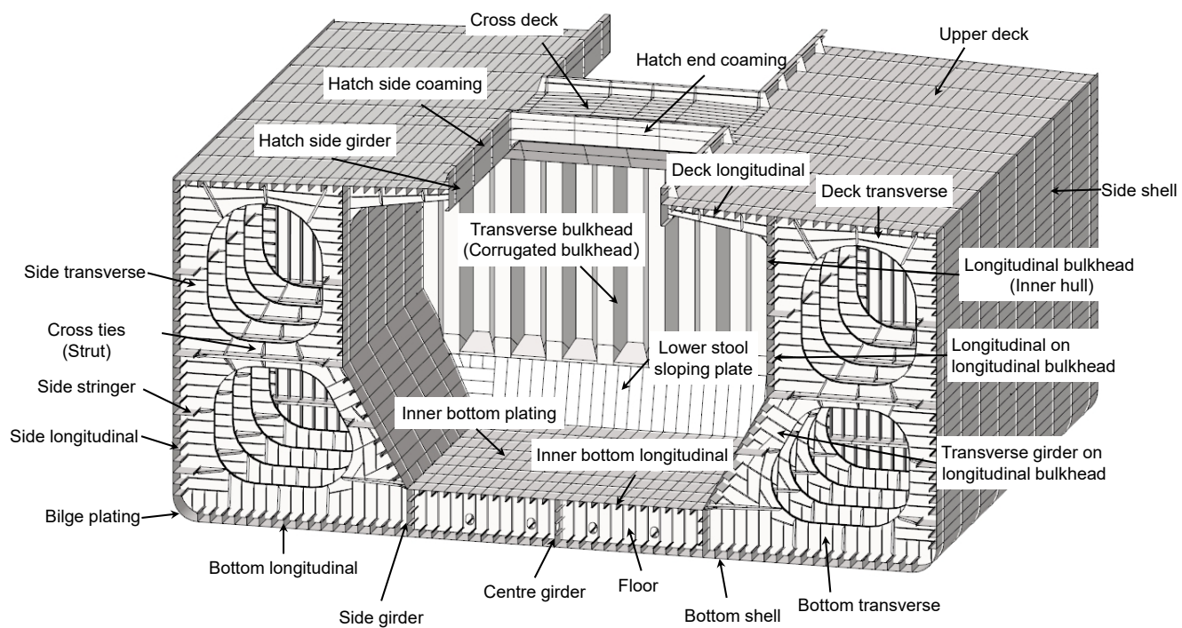
Fig. 1.2.1-1 Ore Carriers
