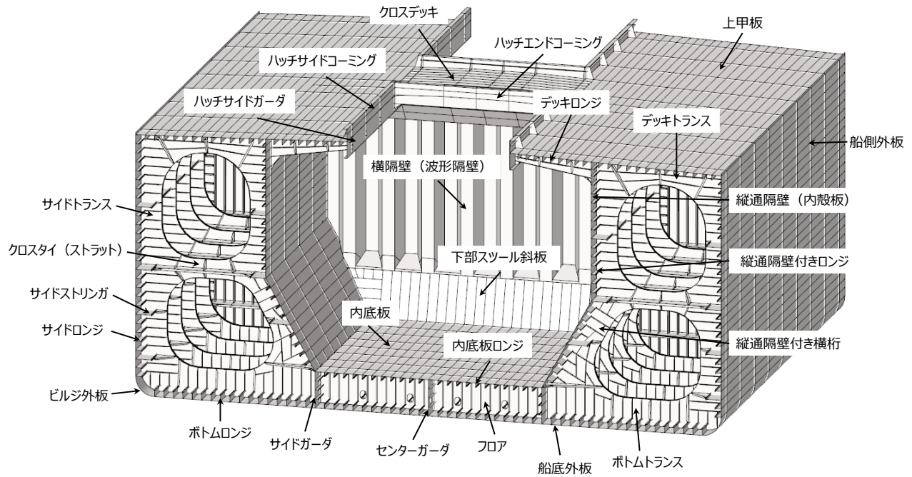
図 1.2.1-1. 鉱石運搬船
