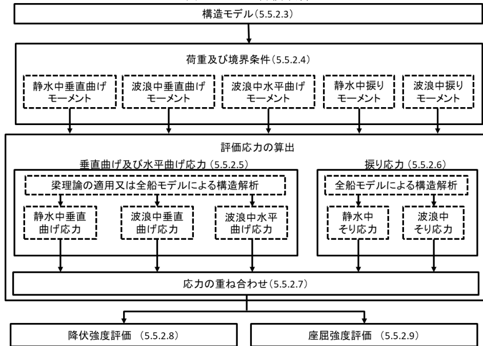
図 5.5.2-1. 評価手順
