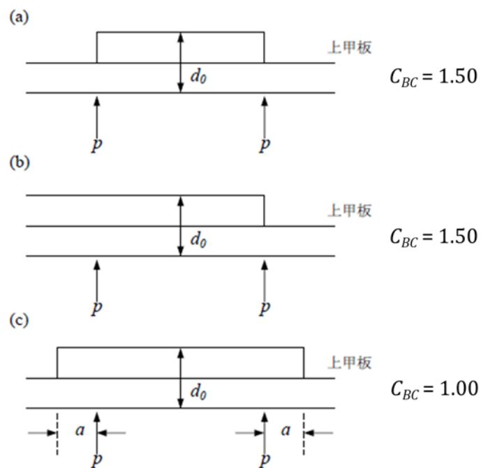
図 7.2.1-1. ピラー等に支持されるハッチサイドガーダ
